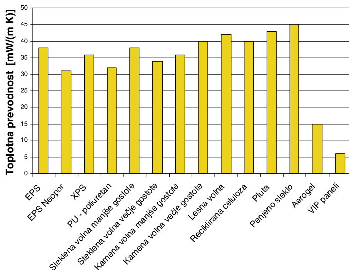
Slika 3 • Vrednosti toplotne prevodnosti (λ) za različne toplotno izolacijske materiale, izražene v mW/(m K)
