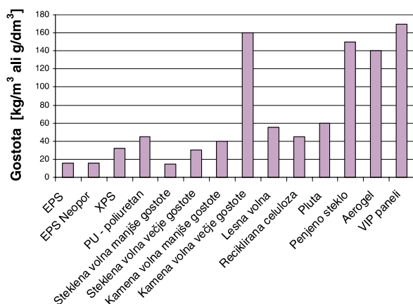
Slika 2 • Gostote različnih toplotnoizolacijskih materialov
