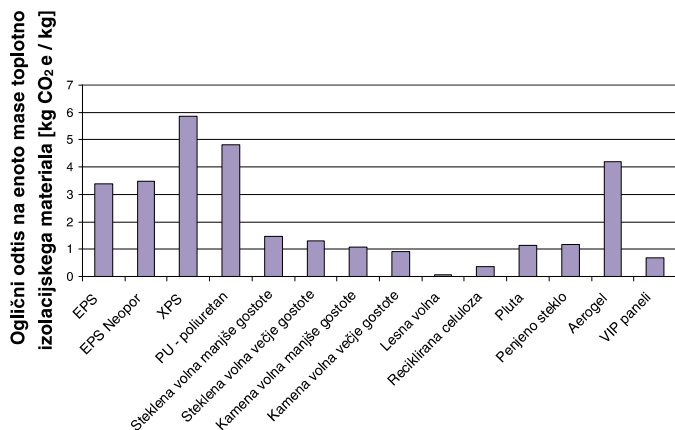
Slika 1 • Ogljični odtis različnih toplotnoizolacijskih materialov, izražen na kilogram mase izbranega materiala
