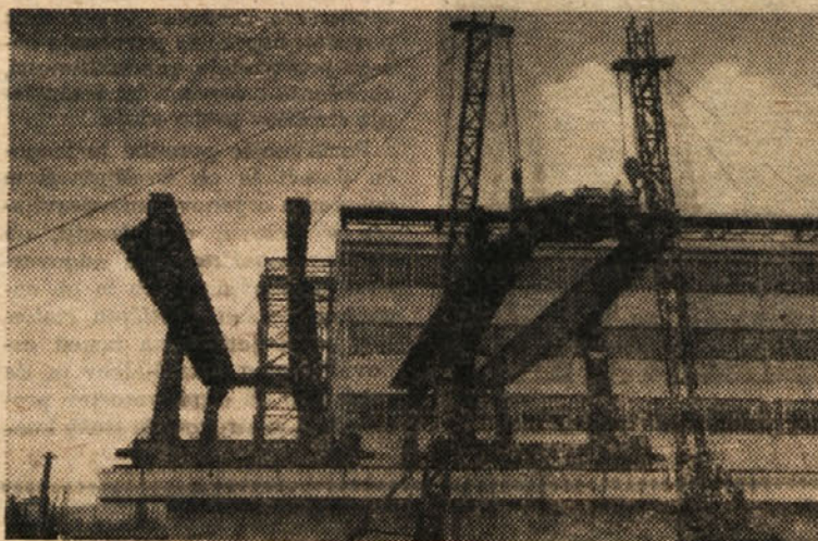
Montaža tekalnega žerjava na rudnem dvoru ob novem obratu žveplene kisline.
