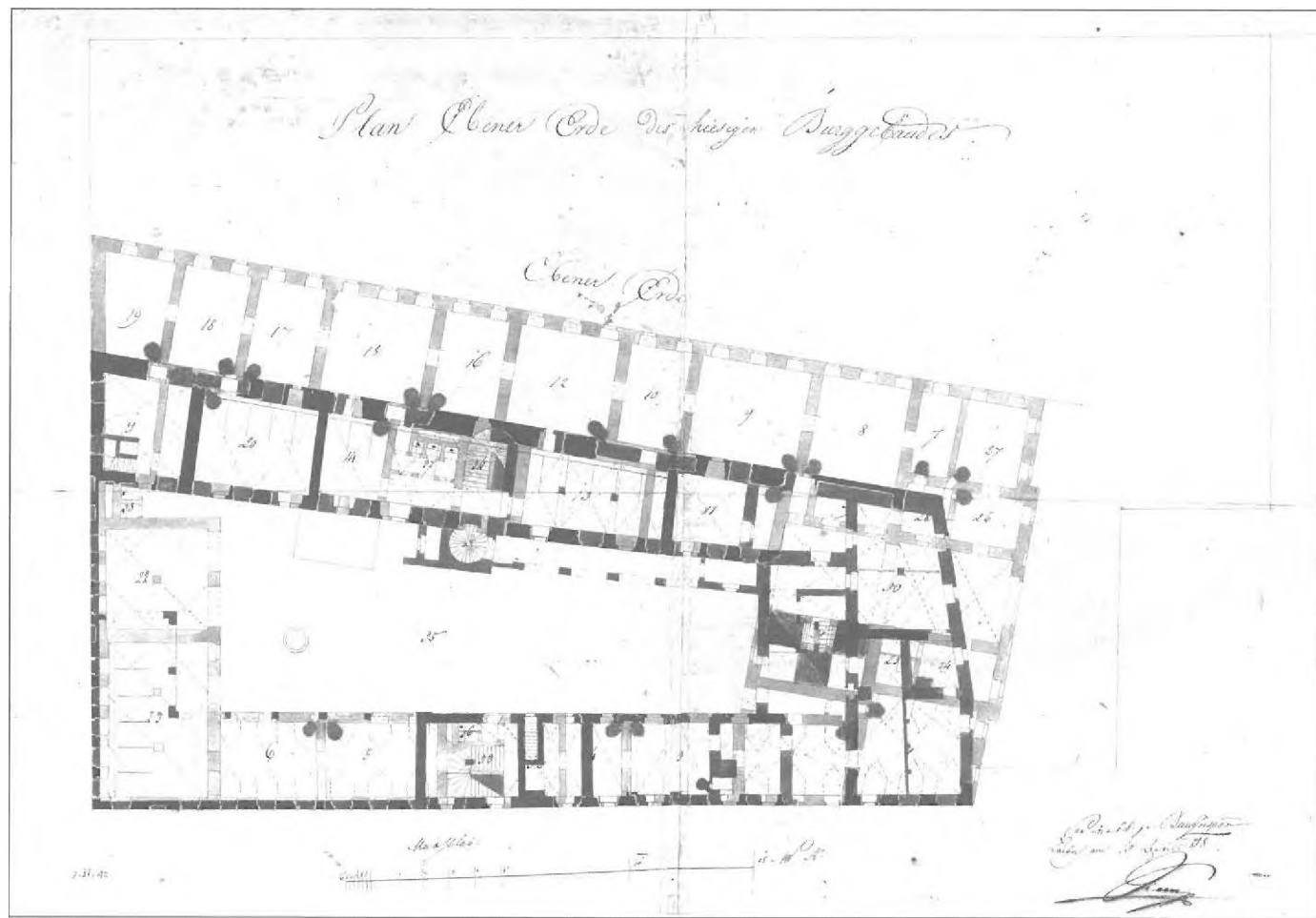
20 Gradbena inšpekcija, Deželni/Vicedomski dvorec na Kongresnem trgu 12, 1828, tloris pritličja, adaptacija in dozidava, kolorirana matrica / 64 x 45; ZAL, Načrti (LJU 334), mapa 10/9, 1
