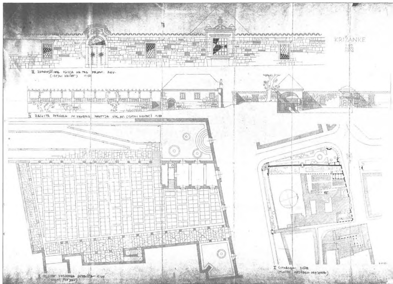
24 Seminar Jožeta Plečnika, Križanke na Trgu francoske revolucije 2, 1952, zid na Trgu francoske revolucije, razvita pergola in vhodna partija velikega dvorišča, tloris velikega dvorišča, situacija, idejni načrt, kopija / 94 x 66,9; ZAL, Mestni ljudski odbor Ljubljana, komunala in gradnje (LJU 474)
