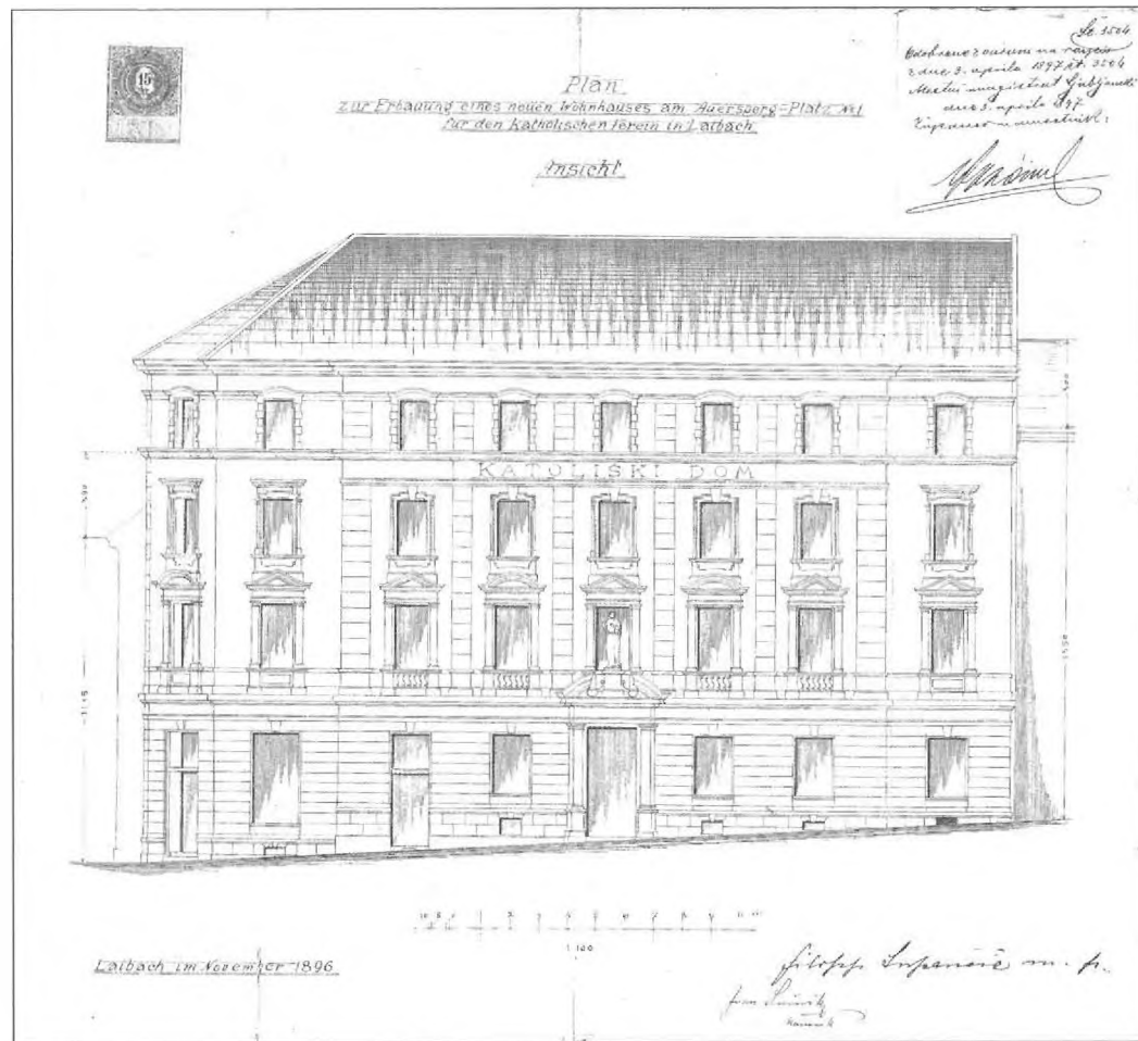
21 Katoliški dom na Novem trgu 1, 1896 , fasada, gradnja zgornjega nadstropja, kopija / 38,6 x 35,7; ZAL, Mesto Ljubljana, splošna mestna registratura (LJU 489), Reg I, f. 1147, fol. 62
