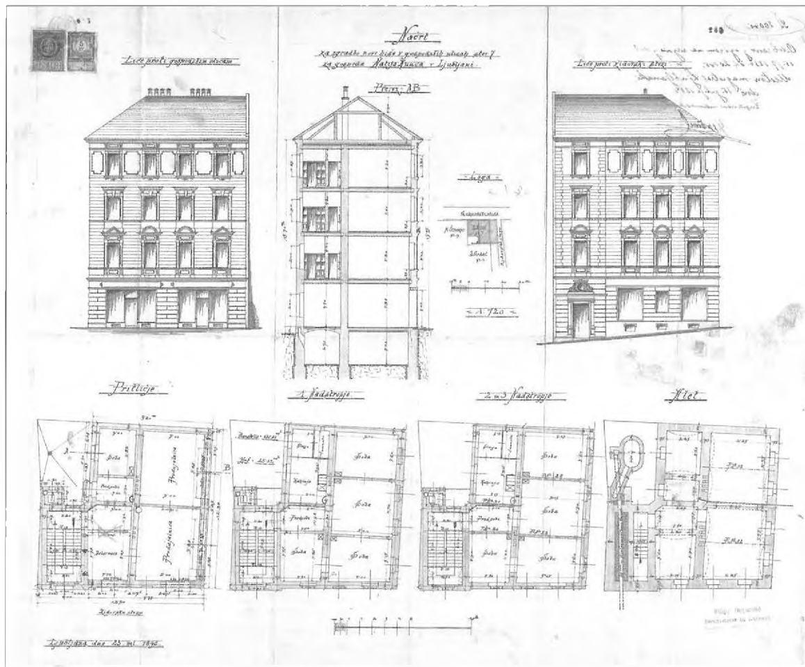
16 Stanovanjska hiša na Židovski stezi 2 (Gosposki ulici 7), 1896, fasadi, prerez, situacija, tlorisi etaž, gradnja/adaptacija, kolorirana matrica / 64,4 x 54; ZAL, Mesto Ljubljana, splošna mestna registratura (LJU 489), Reg I, f. 1145, fol. 682
