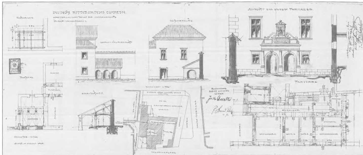
23 Komenda nemškega viteškega reda/Križanke na Trgu francoske revolucije 1 (Gosposka ulica), 1905, delna tlorisa ostrejša in pritličja, prerez verande, fasadi na vrtni strani, situacija, del vhodne fasade in tloris dela pritličja, adaptacija, kolorirana kopija / 84,3 x 35,4; ZAL, Mesto Ljubljana, splošna mestna registratura (LJU 489), Reg I, f. 1153, fol. 115
