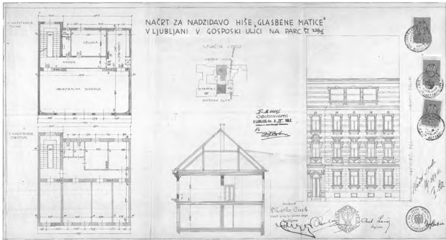
13 Josip Platner, Glasbena matica v Gosposki ulici 8, 1933, tlorisa 2. in 3. nadstropja, situacija, prerez, fasada, nadzidava, kolorirana kopija / 63,4 x 33,8; ZAL, Mesto Ljubljana, gradbena registratura (LJU 493), Reg IV
