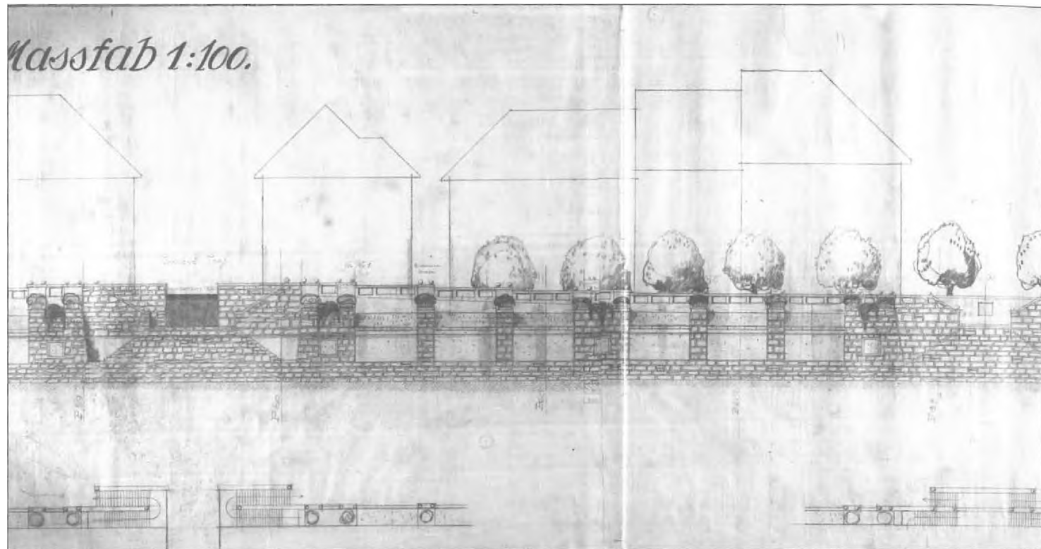
9 Alfred Keller, Regulacijski načrt obrežnega zidovja Ljubljane med Jučičevim trgom in filharmonijo, 1913, pogled in delni tloris, detajl, kolorirana matrica / 525 x 57,1; ZAL, Načrti (LJU 334), mapa 01/4, 5
