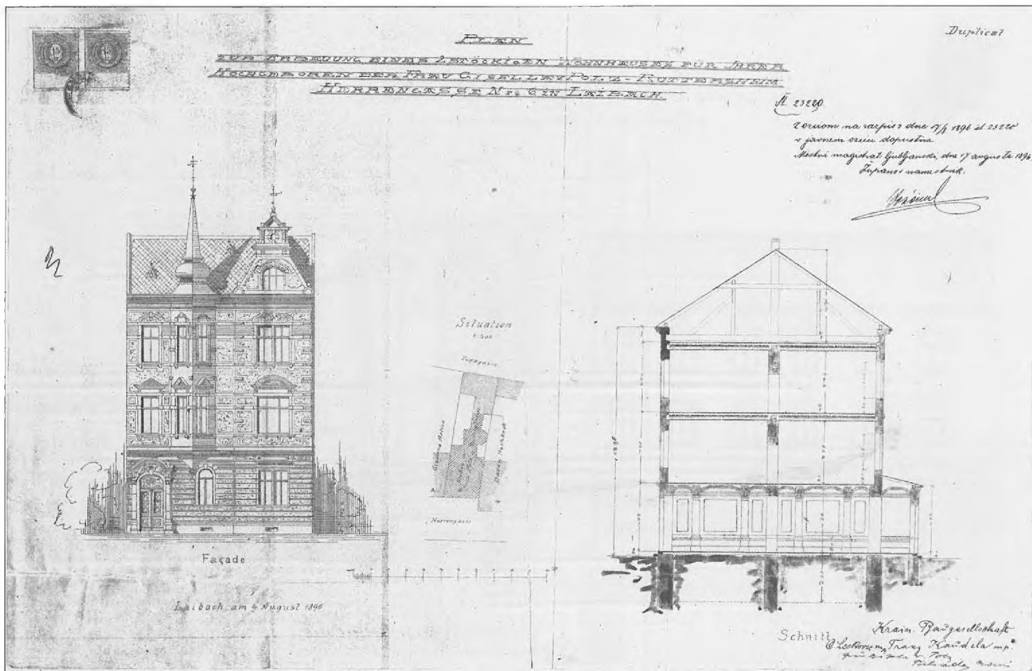
12 Stanovanjska hiša v Gosposki ulici 6, 1896, fasada, situacija, prerez, gradnja 2. nadstropja, kolorirana kopija / 57,6 x 37,1; ZAL, Mesto Ljubljana, splošna mestna registratura (LJU 489), Reg I, f. 1144, fol. 577
