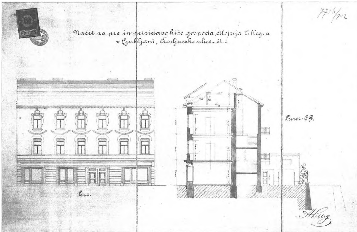
11 Stanovanjska hiša v Čevljarški ulici 3, 1902, glavna fasada, prerez, adaptacija (podrta 1914–1918), kolorirana kopija / 53,6 x 33,7; ZAL, Mesto Ljubljana, splošna mestna registratura (LJU 489), Reg I, f. 1511, fol. 183
