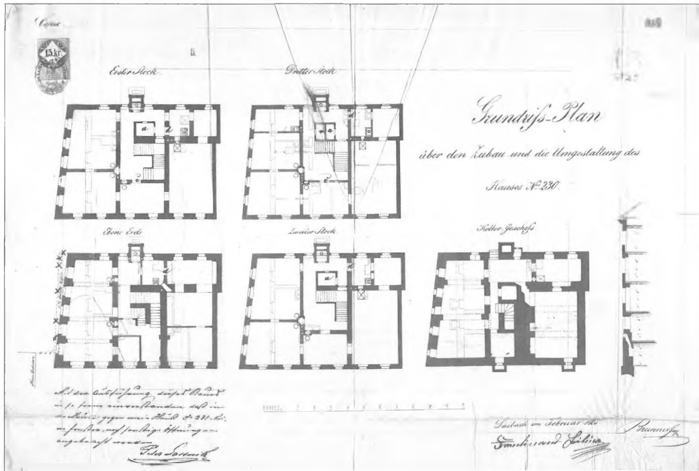
17 Brunner, Stanovanjska hiša v Židovski ulici 1, 1865, tlorisi etaž, delni prerez, adaptacija, kolorirana matrica / 54,9 x 36,5; ZAL, Mesto Ljubljana, splošna mestna registratura (LJU 489), Reg I, f. 753, fol. 240
