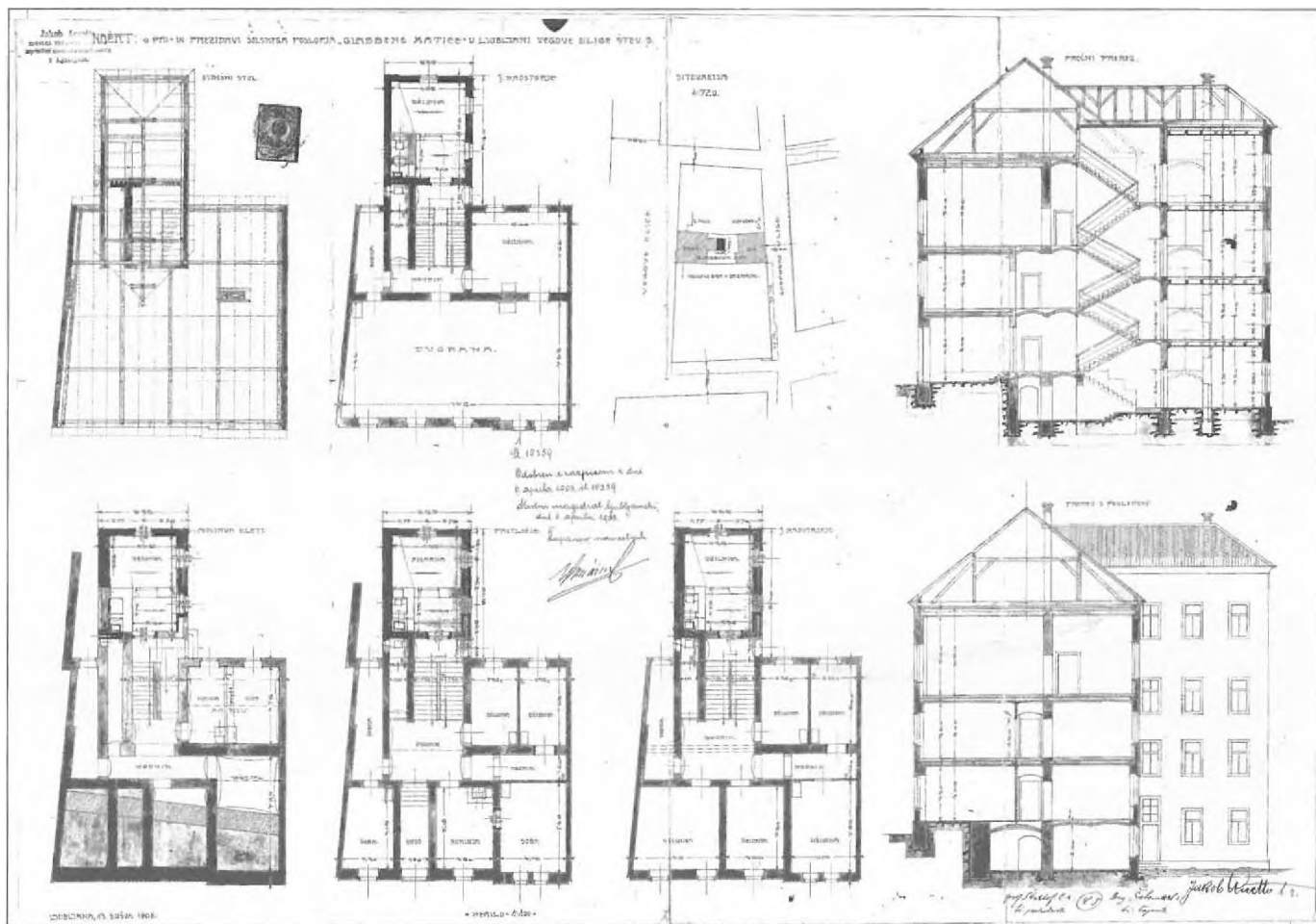
15 Glasbena matica v Vegovi ulici 7, 1908, tlorisi etaž, situacija, prerez, prerez z dvoriščno fasado, adaptacija šolskega posloppja in gradnja prizidka, kolorirana kopija / 81,4 x 56,6; ZAL, Mesto Ljubljana, splošna mestna registratura (LJU 489), Reg I, f. 1532, fol. 234
