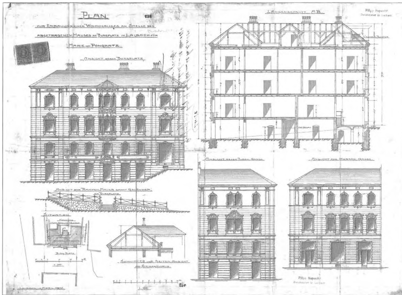
18 Stanovanjska hiša na Dvornem trgu 2, 1896, fasade, prereza, situacija, pogled na ograjo, gradnja zgornjega nadstropja, kolorirana matrica / 68,2 x 50,3; ZAL, Mesto Ljubljana, splošna mestna registratura (LJU 489), Reg I, f. 1144, fol. 342
