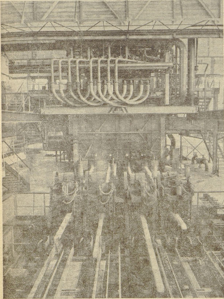
Konti naprava med odlivanjem jekla
