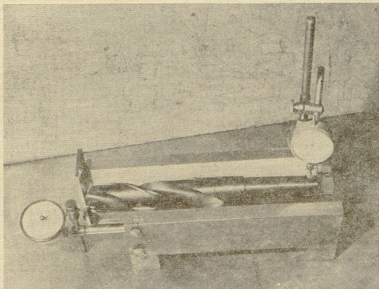
Naprava za kontrolo spiralnih svedrov. Avtorja: Omerzu Mihael, Milanović Slobodan
