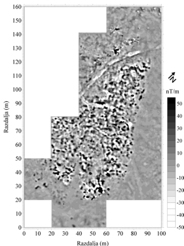
Sl. 39: Branževce nad Seli pri Dolenjskih Toplicah. Železarski talilniški prostor. M. = 1: 1000 (po Mušič, Orengo (op. 41)). Abb. 39: Branževce bei Sela pri Dolenjskih Toplicah. Vchüttungsplatz. M. = 1: 1000 (nach Mušič, Orengo (Anm. 41)).
