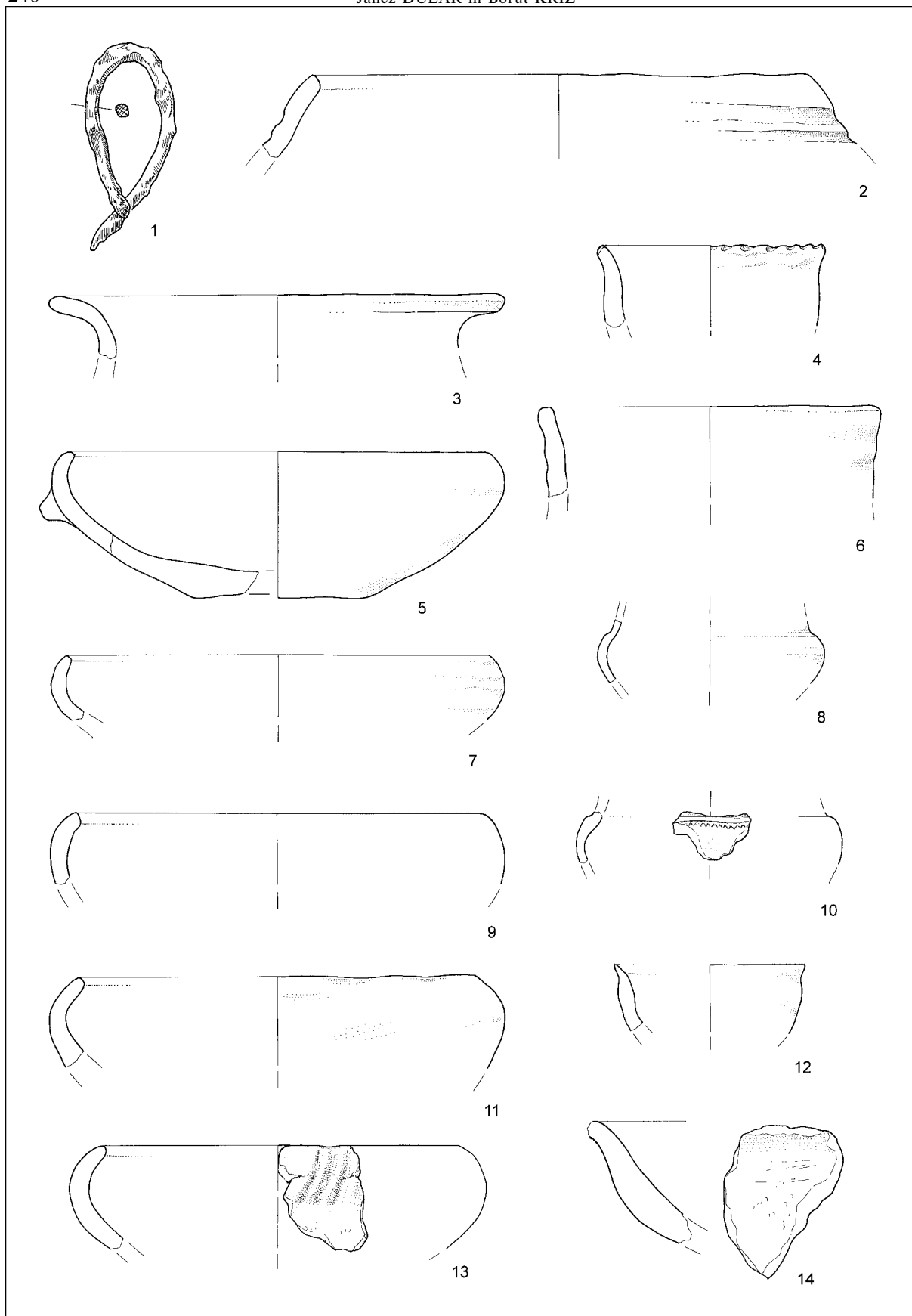
T. 8: Sonda 3. 1-14 plast 6. 1 železo, ostalo keramika. M. 1= 1:2; 2-14 = 1:3.
