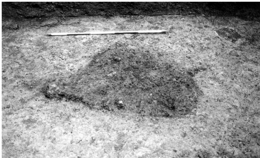
Sl. 38: Branževce nad Seli pri Dolenjskih Toplicah. Talilna peč 4. Abb. 38: Branževce bei Sela pri Dolenjskih Toplicah. Rennofen 4.
