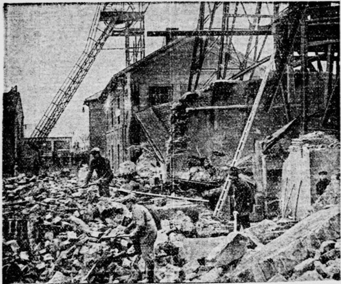
Odstranjevanje razvalin okoli šahta, katerega nadzemske naprave so bile zaradi podzemne eksplozije docela uničene.
