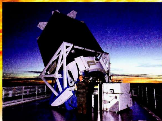
Teleskopi vsake toliko časa odkrijejo novo nebesno telo.
