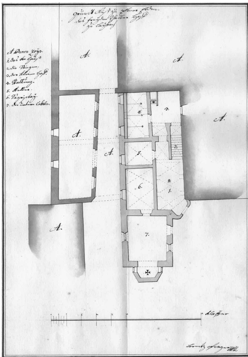
Lovrenc Prager, Bistriški dvor, tloris pritličja, 1790, vir: StLA, FLD, Staatsguterakten Krainerische Archivalien, Versch. H. Freudenthal (5. Theil), Karton 96.
