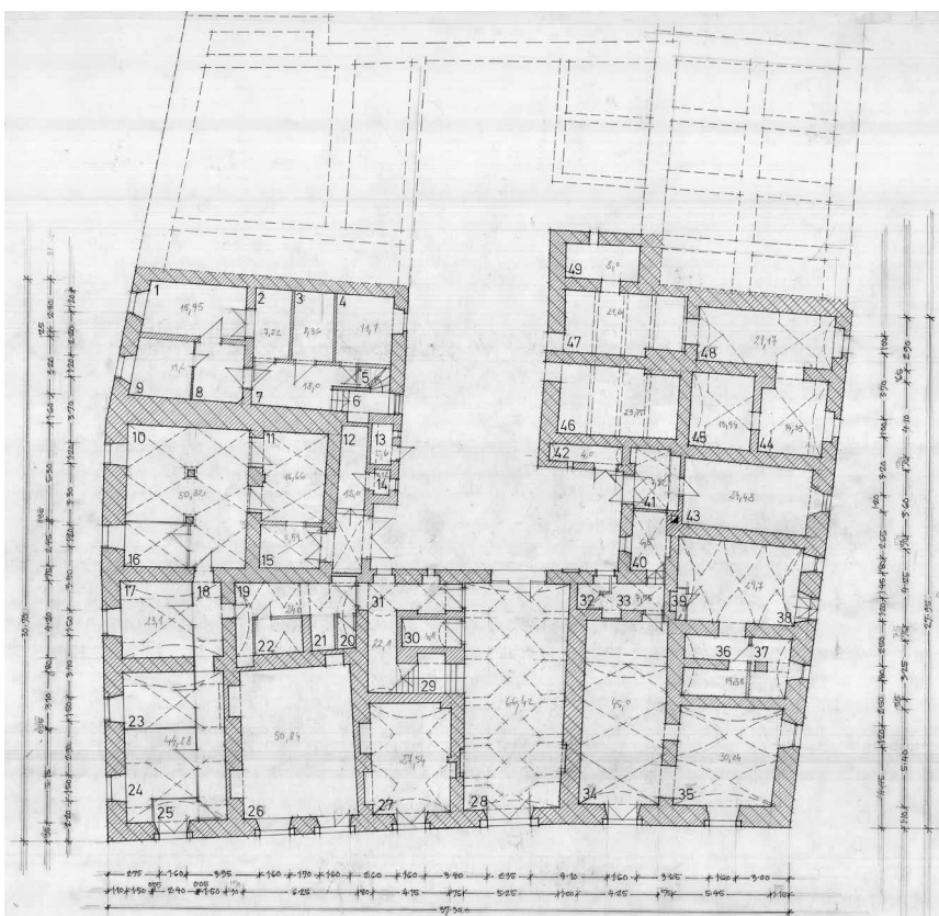
Zoisova palača, tloris pritličja, vir: ZVKDS, M. Stražišar, 1982
