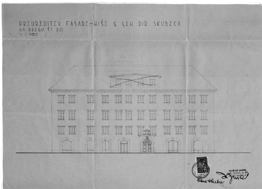
Načrt prezidave Zoisove palače, fasada, 1932, vir: SI ZAL, LJU 493-Reg-IV-B-TE27
