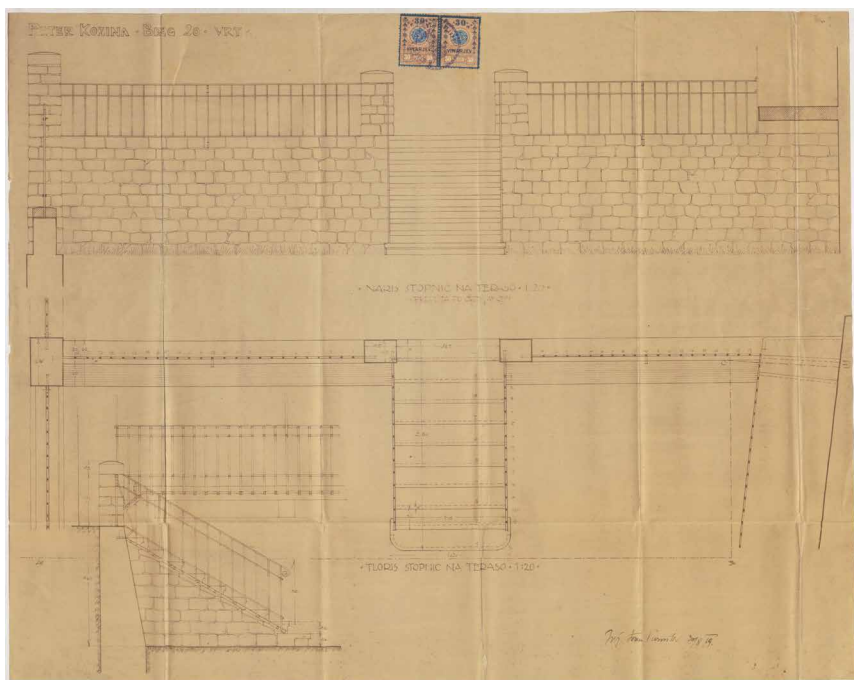
41. Ivan Vurnik, Načrt ograje, Načrt ograje, 1919, SI ZAL, Reg I., LJU 489, fasc. 1789
