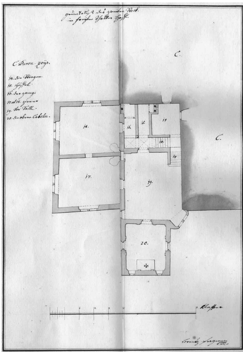
Lovrenc Prager, Bistriški dvor, tloris drugega nadstropja, 1790, vir: StLA, FLD, Staatsguterakten Krainerische Archivalien, Versch. H. Freudenthal (5. Theil), Karton 96.
