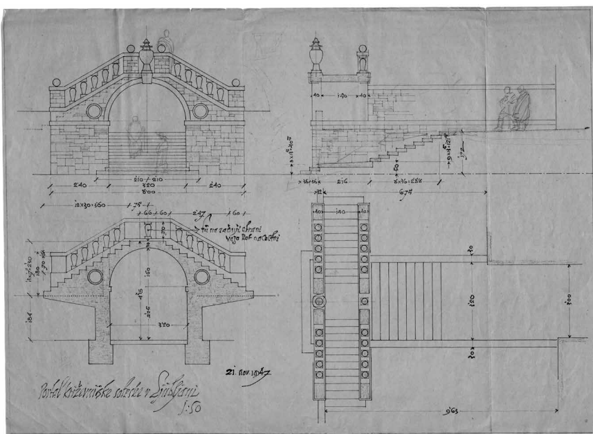
Jože Plečnik, načrt prehoda iz Križevniške soteske na Zoisovo cesto, 1947, SI ZAL, LJU, MLO Ljubljana 474/2, 009, 5171, načrt-portal.
