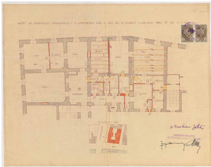
42. Načrt prezidave Zoisove palače, drugo nadstropje, 1932, SI ZAL, LJU, 493-Reg-IV-B-TE27
