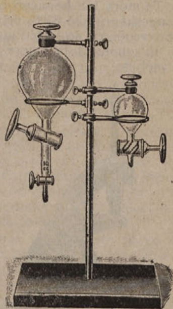
Avtomatična priprava za pipetiranje. Z obračanjem ventilov odmerimo določeno količino žveplene kisline in anilovega alkohola ter spustimo v tolašcomer.
