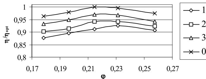
Sl. 3. Diagram izkoristka za nominalno tlačno število \psi=1,011
