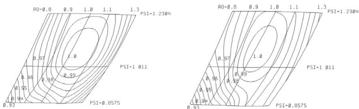
Sl. 4. Školjčna diagrama izkoristka na temelju izračunanih in izmerjenih vrednosti v 15 točkah
