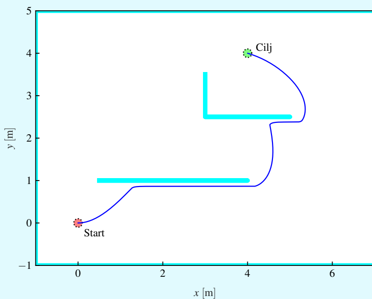
Slika 4.25: Načrtovanje poti in vodenje z algoritmom Hrošč0 za vožnjo robota do cilja ob izogibanju oviram
