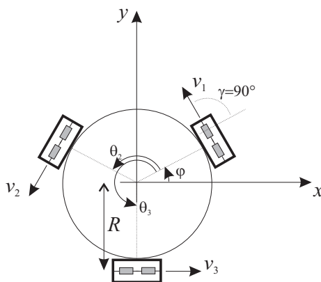
Slika 2.13: Trikolesni večsmerni pogon ( \theta_2 = 120^\circ , \theta_3 = 240^\circ )
