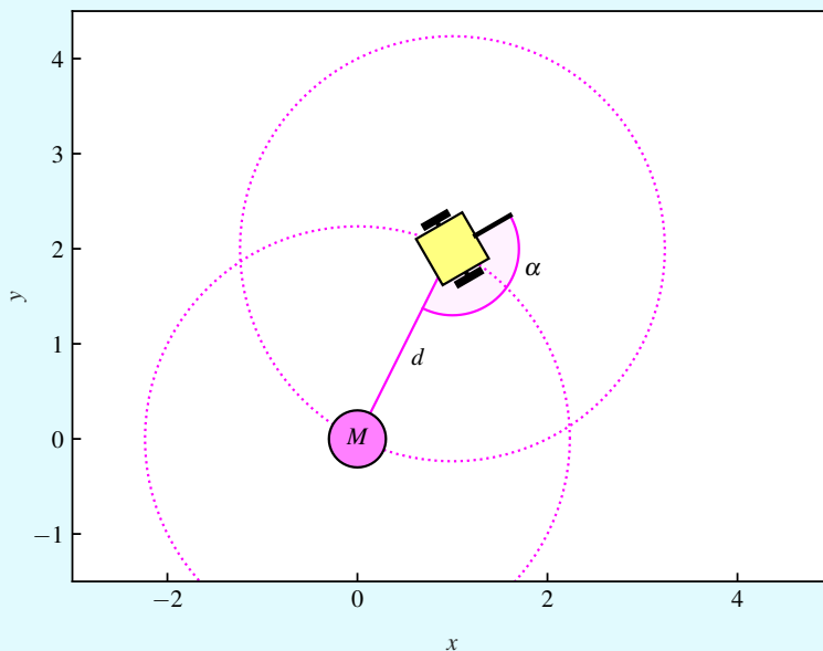
Slika 6.30: Postavitev iz primera 6.21. Mobilni robot ima senzor za merjenje razdalje in kota do značke M , ki se nahaja v izhodišču globalnega koordinatnega sistema.
