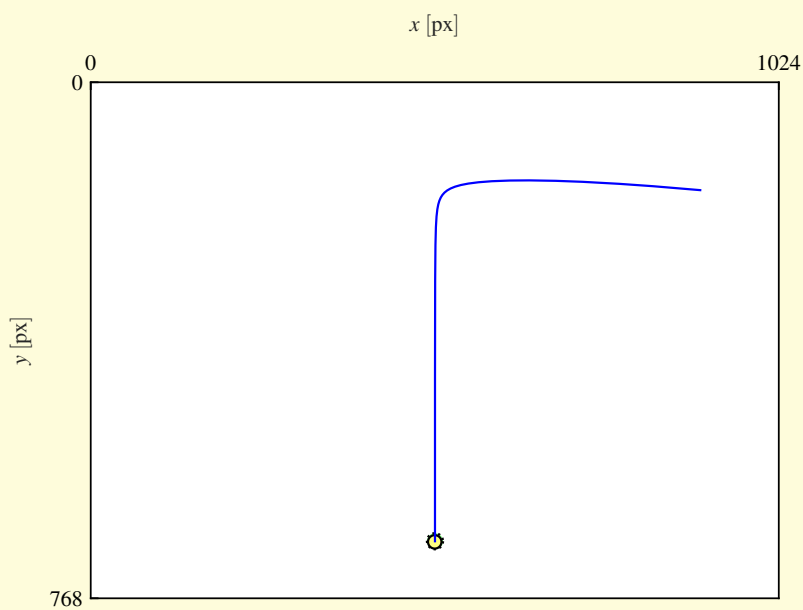
Slika 3.37: Pot opazovane značilke (cilja) v slikovnem prostoru iz primera 3.16
