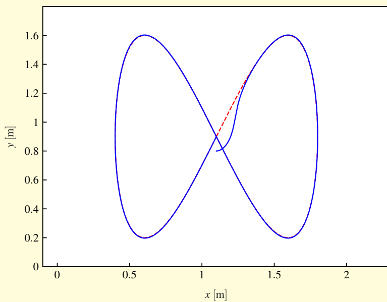
Slika 3.26: Nelinearno vodenje po referenčni trajektoriji vozila z diferencialnim pogonom iz primera 3.11 (referenca je označena s črtkano krivuljo)
