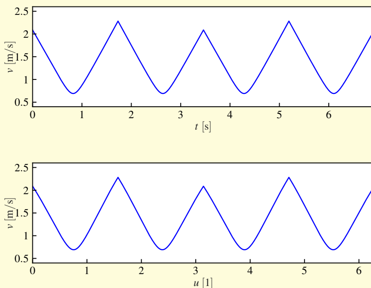
Slika 3.42: Optimalni hitrosti v(u) in v(t)
