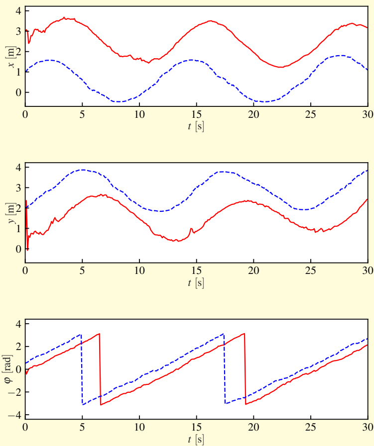
Slika 6.37: Ocena lege (polna krivulja) in pravo stanje (črtkana krivulja) mobilnega robota z začetnim neničelnim pogreškom ocene iz primera 6.21 (reprezentativni primer)
