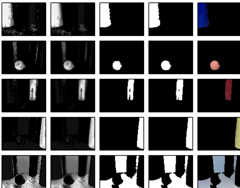
Slika 5.28: Detekcija barvnih značilk. Vsaka vrstica predstavlja drugačno barvo. Koraki od levega do desnega stolpca: povratna projekcija histograma barvne predloge, glajenje, upravljanje, dodatno filtriranje in maskiranje slike
