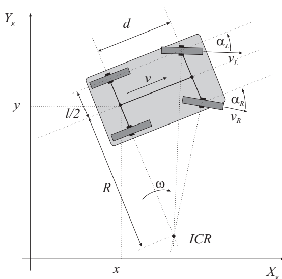
Slika 2.7: Shema Ackermannovega pogona
