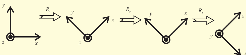
Slika 5.2: Prikaz rotacij z Eulerjevimi koti (5.14)
