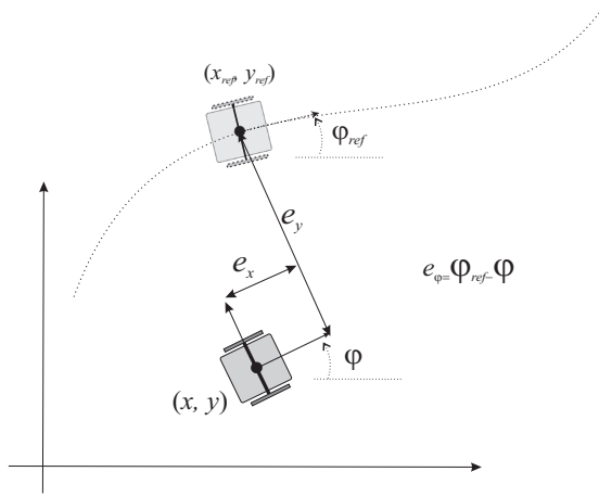
Slika 3.21: Prikaz pozicijskega pogoška v lokalnih koordinatah
