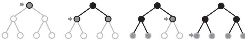
Slika 4.26: Algoritem iskanja v širino najprej razišče najbližja vozlišča. Trenutno vozlišče je označeno s puščico, odprta (živa) vozlišča so označena s svetlo sivimi, zaprta (mrtva) vozlišča s črnimi in nepreverjena vozlišča z belimi krogi.
