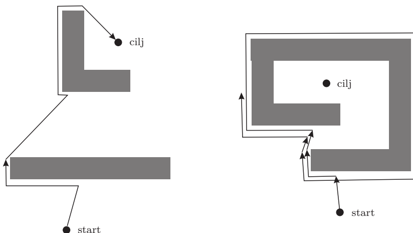
Slika 4.22: Algoritem Hrošč0 (varianta vedno zavij levo) uspešno najde pot do cilja (leva slika) in neuspešno (desna slika)
