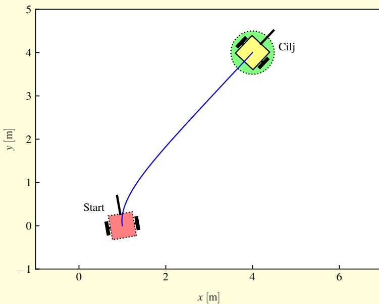
Slika 3.36: Pot pridobljena z IBVS iz primera 3.16
