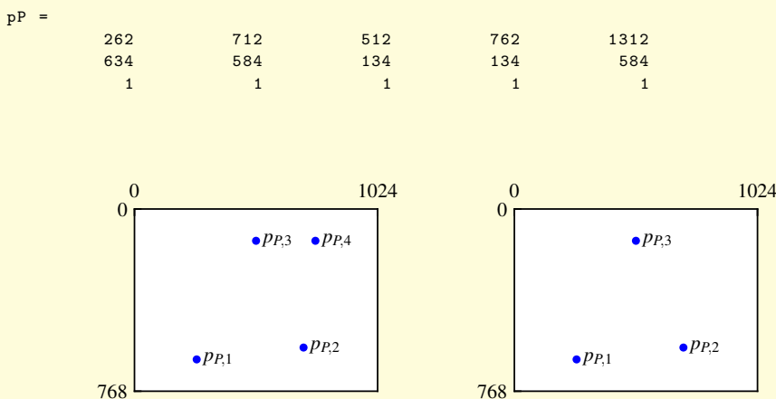
Slika 5.5: Projicirane točke na slikovno ravnino iz primera 5.4. Na levi so točke, ki so preslikane z matematičnim modelom (5.24) in na desni so točke, ki so v resnici vidne na slikovni ravnini.
