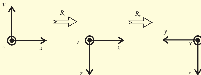
Slika 5.3: Prikaz rotacije (5.15)
