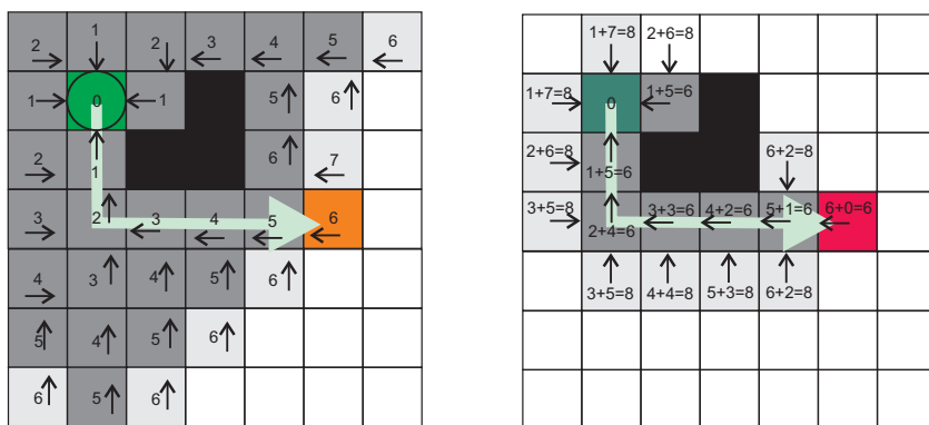
Slika 4.31: Primerjava algoritmov iskanja poti: Dijkstrov (levo) in A* (desno). Oba najdeta najkrajšo pot do cilja, vendar A* porabi precej manj iteracij zaradi uporabe dodatne informacije (hevristike) pri iskanju poti.
