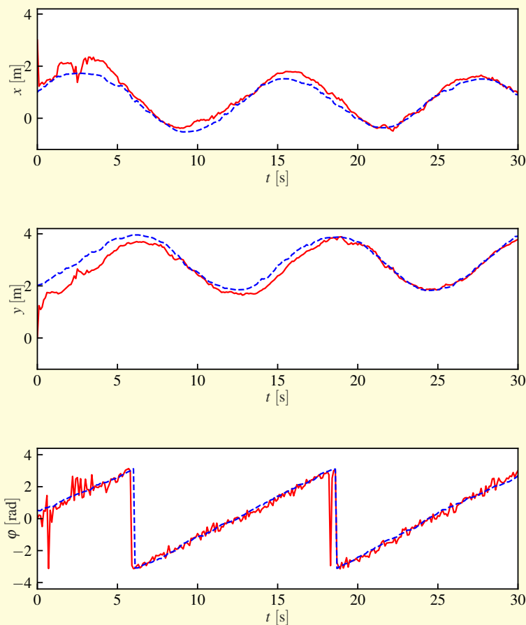
Slika 6.53: Ocena lege (polna krivulja) in pravo stanje (črtkana krivulja) mobilnega robota z začetnim neničelnim pogreškom ocene iz primera 6.24
