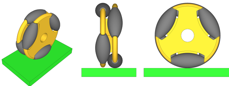
Slika 2.10: Kolo omni s šestimi “prostovrtečimi” se valjčki, ki so razporejeni po obodu kolesa. Kolo se lahko vrti in bočno drsi (vrtijo se valjčki).
