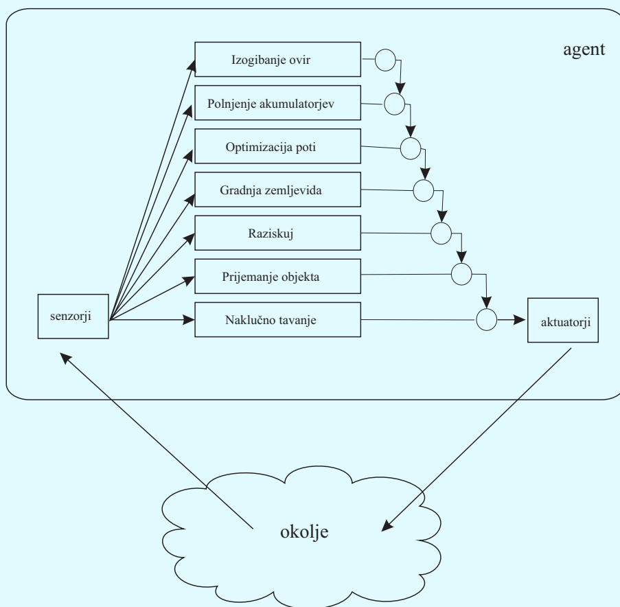
Slika 7.7: Vsebovana shema
