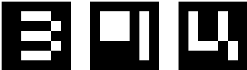
Slika 5.30: Umetne značke
