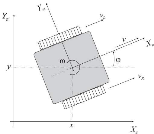
Slika 2.14: Gosenični pogon
