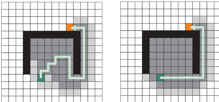
Slika 4.32: Primerjava algoritmov iskanja poti: Pohlepno iskanje najprej-najboljše (levo) in A^* (desno). Pot, ki jo najdemo s pohlepnim iskanjem na način najprej najboljše, ni vedno optimalna. Odrpna vozlišča so označena s svetlo sivo, zaprta vozlišča pa s temno sivo.
