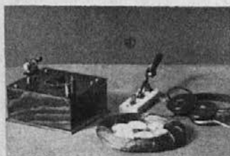
Kompleten detektorski aparat, kakršne oddaja Radio Ljubljana brezplačno novim naročnikom.
