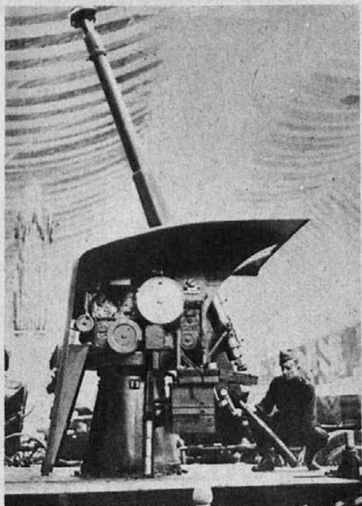
Najnovejši avtomatični obrambni top za letala.
