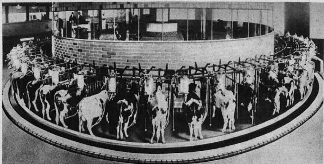
«Rotolaktor», vrteča se plošča, avtomatično umije, posuši in pomolze istočasno 50 krav.
