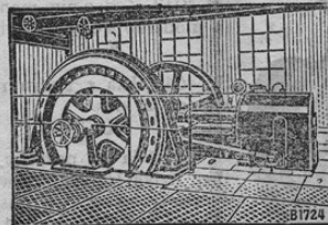
LANZEV ventilni lokomobil za vroči sopar z naravnost pripetim dinamom.
