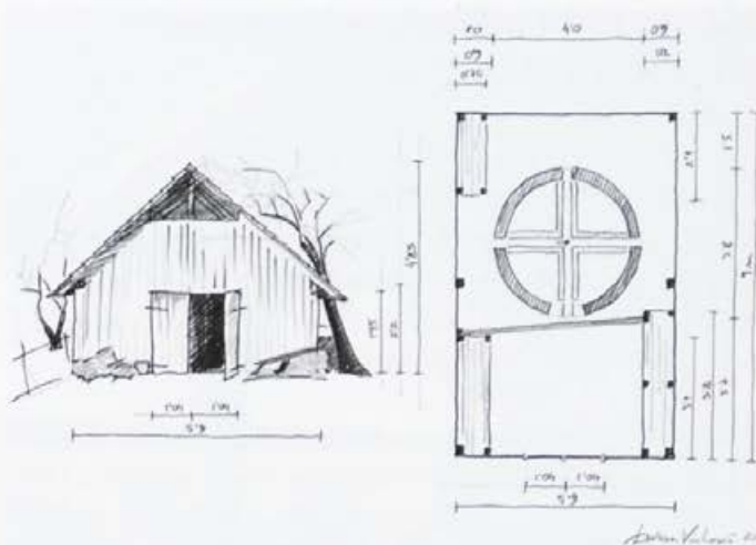
Stavba, v kateri je peč, in tloris peči. Skica: Dušan Vinkovič.
