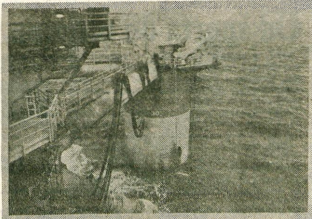
Zagreb I ima pet "nog", ki so 22 metrov potopljene v vodo, na kar morajo nenehno paziti, saj delo na ploščadi poteka noč in dan, vse leto. Delavci delajo neprekinjeno štirinajst dni, po dvanajst ur na dan, nato grdo za štirinajst dni domov.
