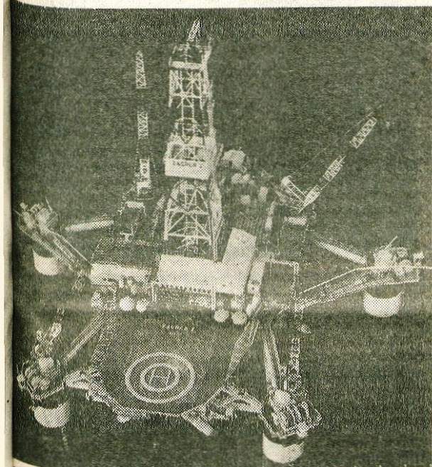
Naftna ploščad Zagreb I je bila leta 1977 zgrajena v francoski ladarnici Dunkerque, stara je torej dvanajst let in najmanj deset let jo še uporabljali. V svetu velja, da se naftna ploščad odplača v približno petih letih, nato pa do petnajst let prinaša dobiček.
