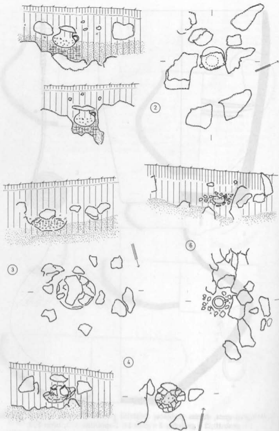
T. 4: Brinjeva gora, žarno grobišče. Profili in tlorisi grobov 2, 3, 4, 6. M 1 : 20. Taf. 4: Brinjeva gora, Urnengräberfeld. Profile und Grundrisse der Gräber 2, 3, 4, 6. M 1 : 20.
