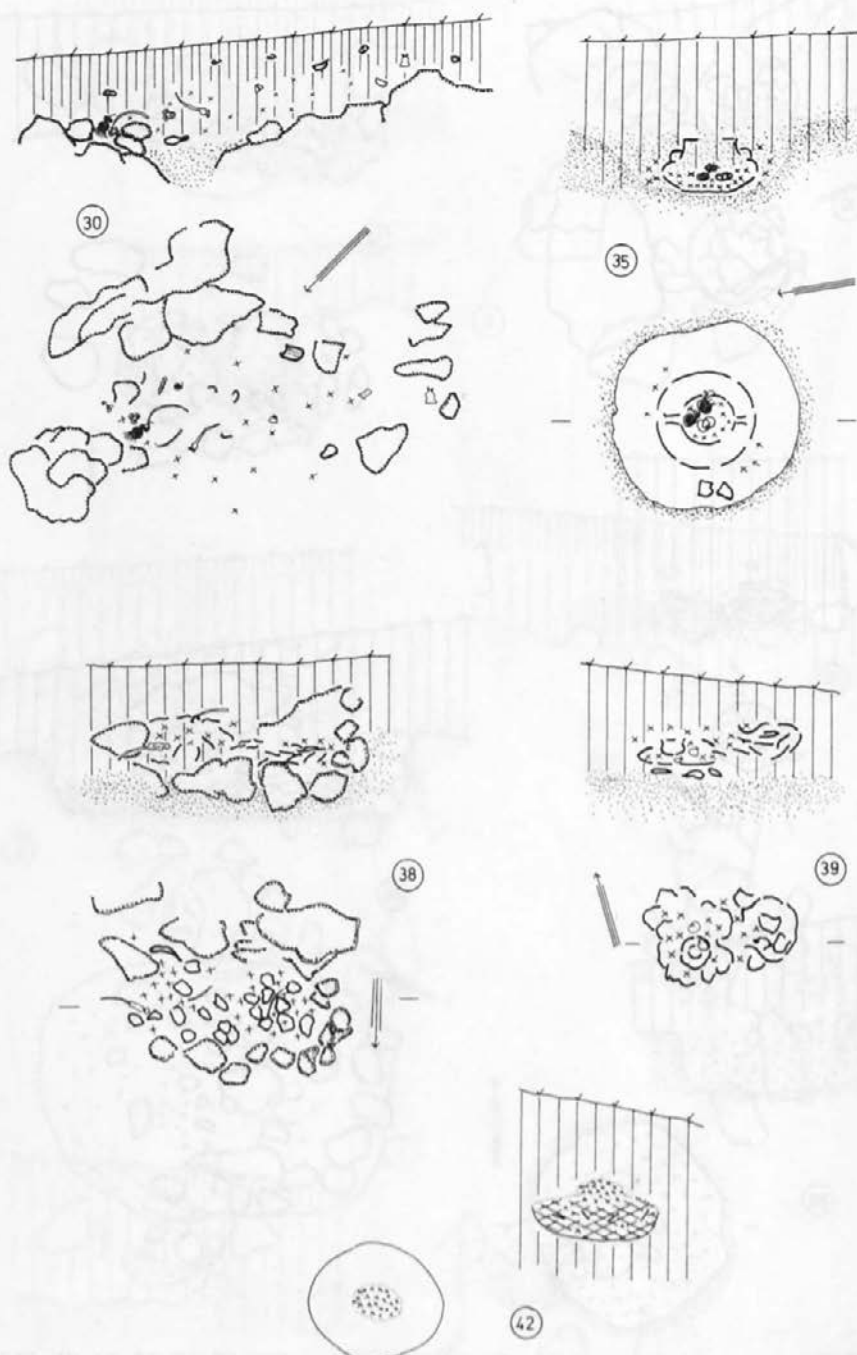
T. 6: Brinjeva gora, žarno grobišče. Profili in tlorisi grobov 30, 35, 38, 39, 42. M 1 : 20.
