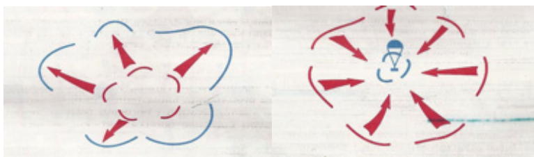
Slika 2: Notranje smeri podiranja
