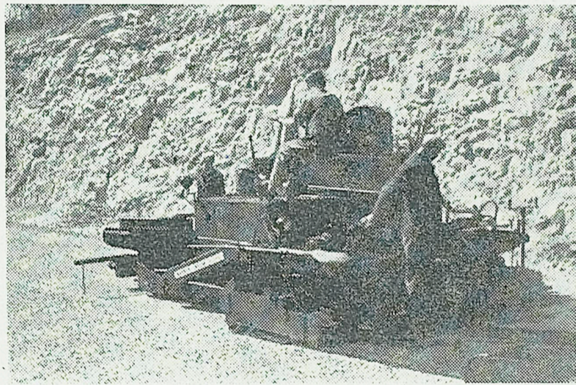
Z naravnost igrivo eleganco polaga finišeer »Barber Green« asfaltno maso na pripravljeno cestišče. Prvi pritisk na podlago opravita dva v stroj vgrajena vibratorja, takoj za njima pa dodobra zvaljajo 170 stopinj C toplo asfaltno maso 3 in 6 tonski valjarji
