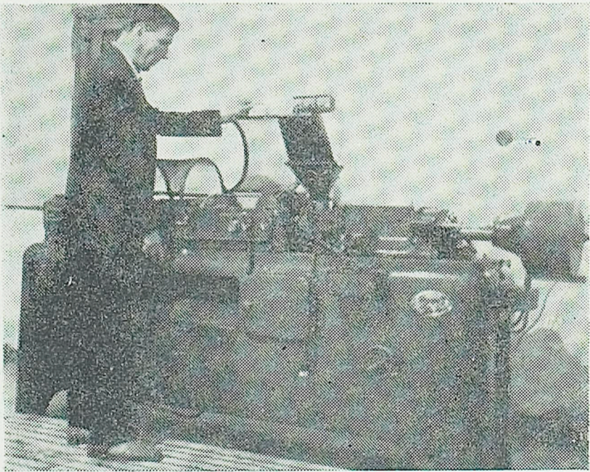
Novi stroj, imenovan injektor (Spritzgussmaschine), za topljenje in vlivanje plastične mase oziroma izdelkov iz te mase, je ponos mladega podjetja Plama, saj mu daje neomejene možnosti za izdelavo zlasti galanterijskih predmetov za široko potrošnjo
