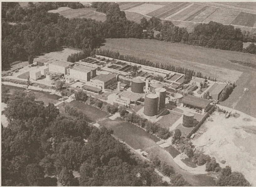
Centralna čistilna naprava Domžale Kamnik bo po rekonstrukciji, ki bo zahtevala dve milijardi tolarjev, s tehnologijo biofilma ena najsodobnejših v državi.
