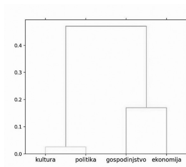
Graf 5: Hierarhično gručenje vektorskih reprezentacij besed na primeru podkorpusev besedil z visoko stopnjo kanoničnosti.
