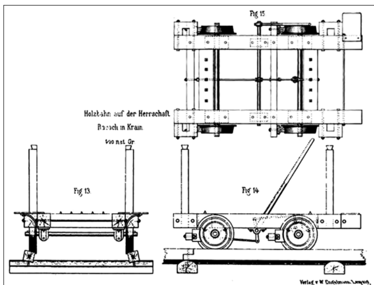
Slika 2: Voziček za prevoz lesa gozdne železnice v dolini Glažute na Jagnjenici pri Radečah
