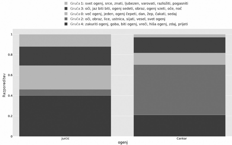
Slika 3: Grafični prikaz pomenskih razlik v rabi leksema ogelj , zaznanih z metodo za zaznavanje semantičnih premikov.
