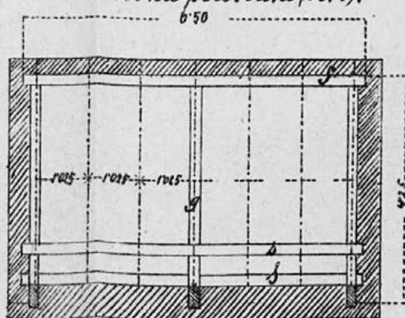
Strešna podstava (očrt).
