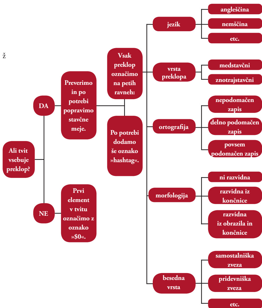
Slika 1: Shema poteka označevanja kodnih preklompov v programu WebAnno.
