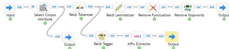
Slika 7: Podproces za obdelavo podkorpsov korpusa komentarjev Evrovizije.
