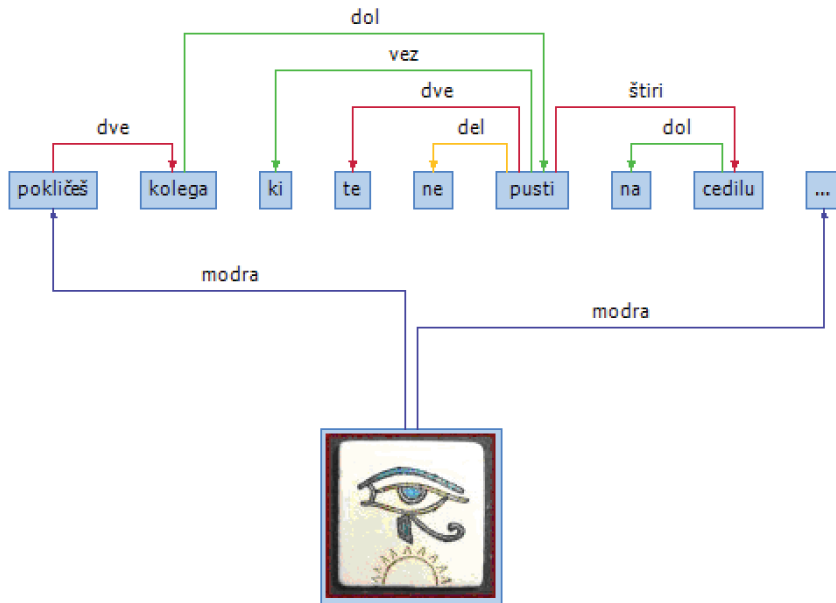
Slika 8: Primer označenega twita v Označevalniku SSJ.
