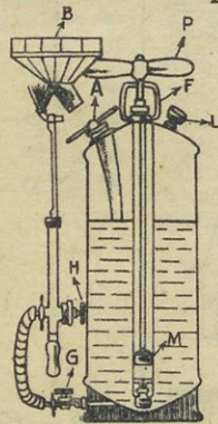
Prerez samodelne škropilnice.
