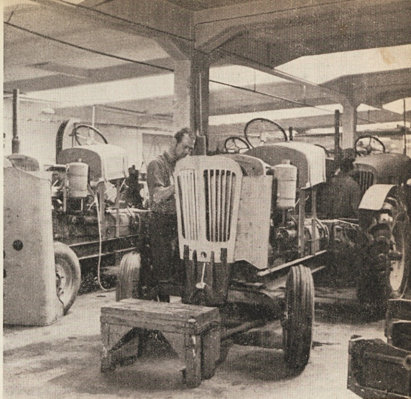
Oddelek znane tovarne motorjev in traktorjev v Rakovici pri Beogradu
