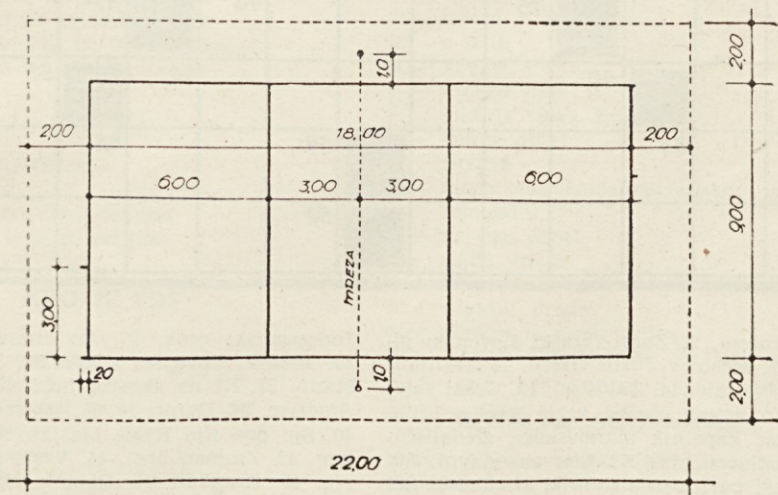
Igrišče za odbojko z merami
