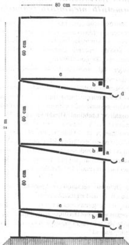
Slika 2. Obris kunčje kletke v prerezu. a) odprtina pod zadnjo steno in med spodnjimi tlemi, b) letva pritrjena na notranjo zadnjo steno, c) zgornja tla, d) žleb za odvajanje moče.
