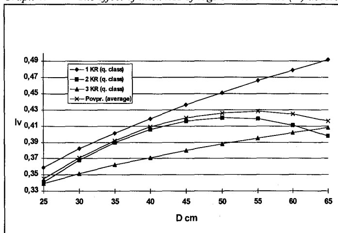
Grafikon 4: Vpliv debeline hlodov na njihovo vrednost ( I_v ) po kakovostnih razredih
