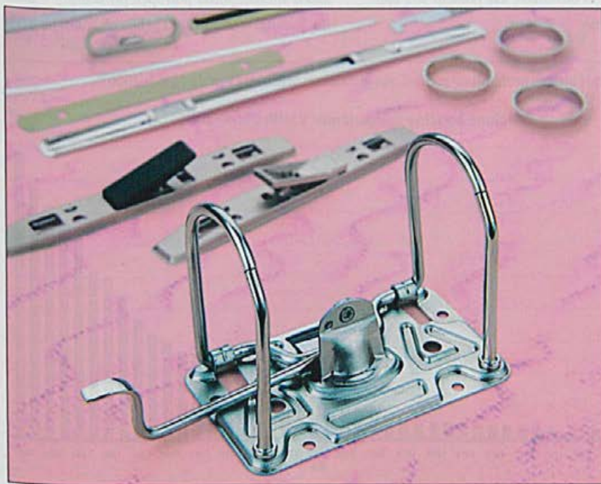
Mehanizem za registrator.
