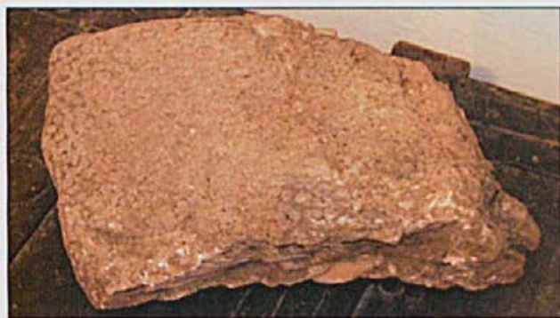
Množica skeletov koralne vrste Waagenophyllum indicum (Waagen et Wentzel) iz zgornjepermijskega apnenca južno od Smoleve pri Železnikih. Foto: Anže Pegam
