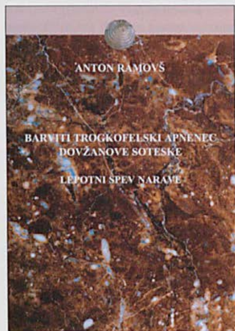
A. Ramovš: Barviti trogkofelski apnencec Dovžanove soteske.
