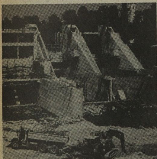
HE Mavčice na Savi pri Kranju naj bi začela poizkusno obratovati v začetku prihodnjega leta
