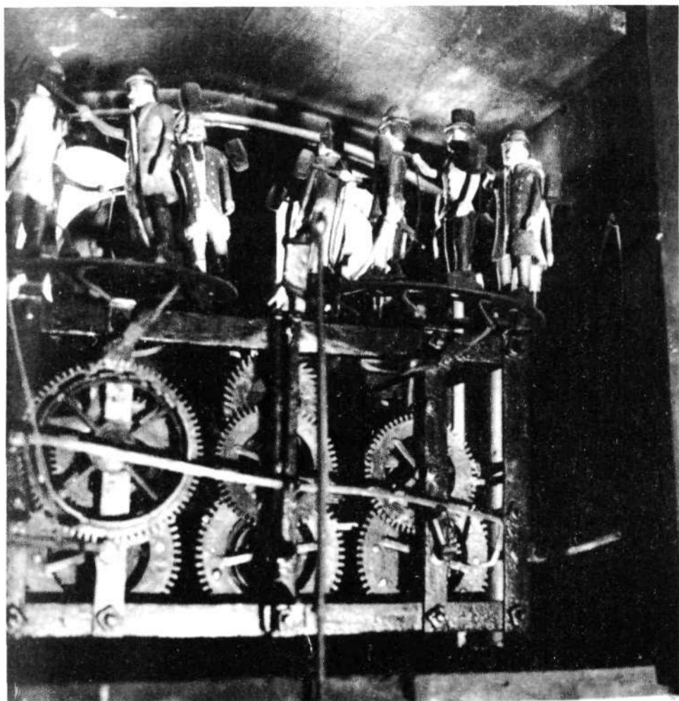
Mehanizem ure s premičnimi figuricami (foto Vesna Bučič)
