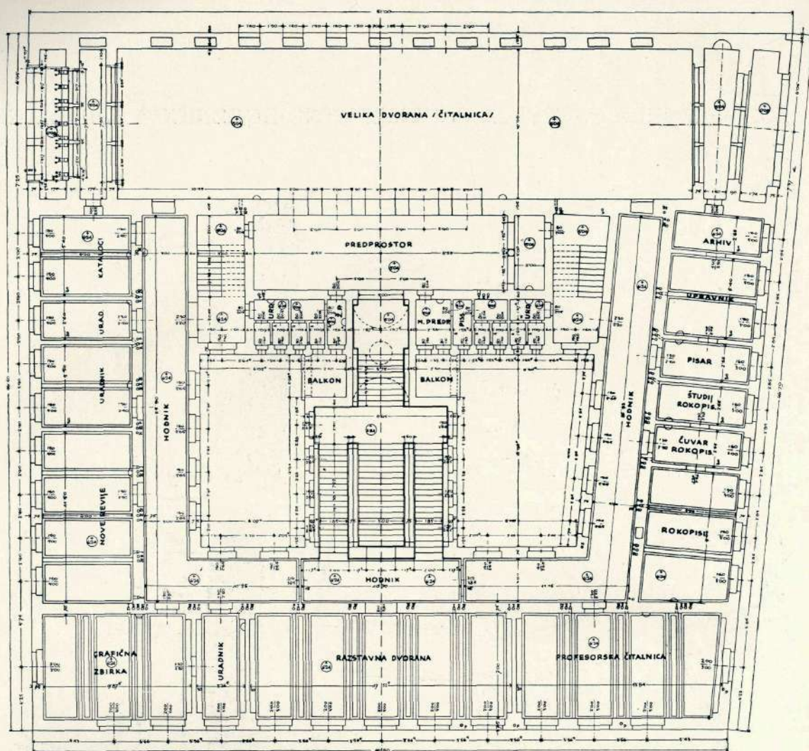
I. NADSTROPJE
