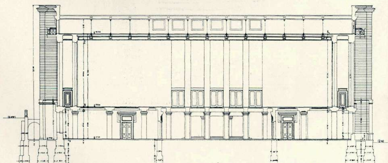
PREREZ A-B
