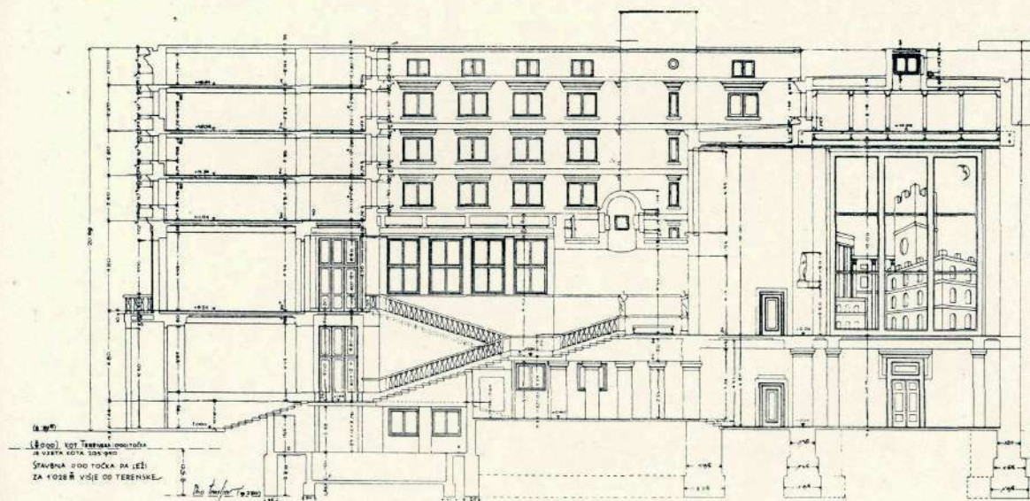
PREREZ C-Č
