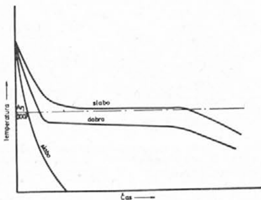
Slika 11 — hitrost ohlajanja Cr-C jekel v odvisnosti od končne temperature — predelave v vročem
