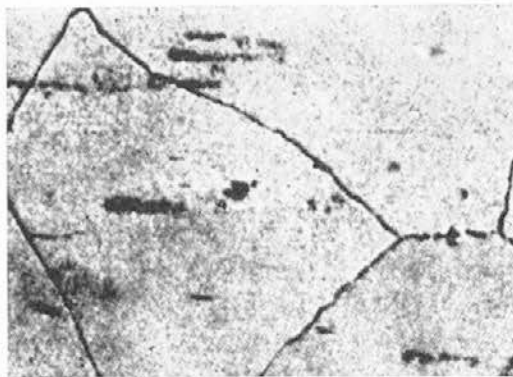
Slika 6 — fina sestava po kovanju 1120 do 1150° C, ohlajevano 75° C/min. Jedkano v natrijevem pikratu, 500 × povečava
