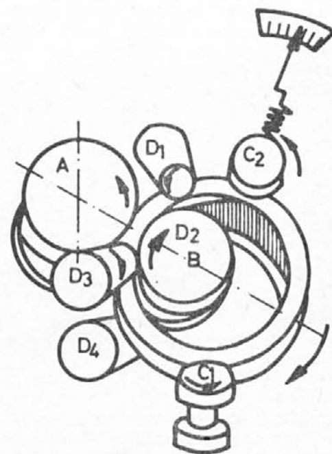
Slika 16 — naprava za profilno valjanje
