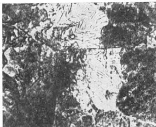
Slika 5 — fina sestava po kovanju pri 1020 do 1050° C, ohlajevano 75° C/min. 500 × povečava
