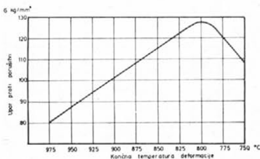
Slika 2 — vpliv preoblikovalne temperature na trdnost kaljenega jekla
