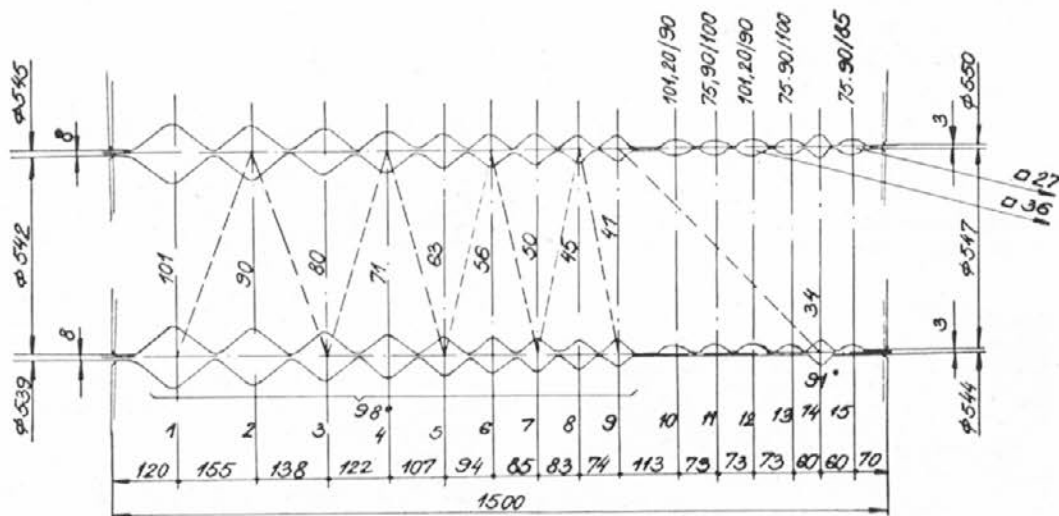
Slika 1 — shema kalibracije II ogrodja
