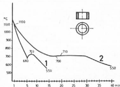
Slika 4 — ohlajevalna hitrost kovanjih ležajev na zraku (1) in v kupu (2)
