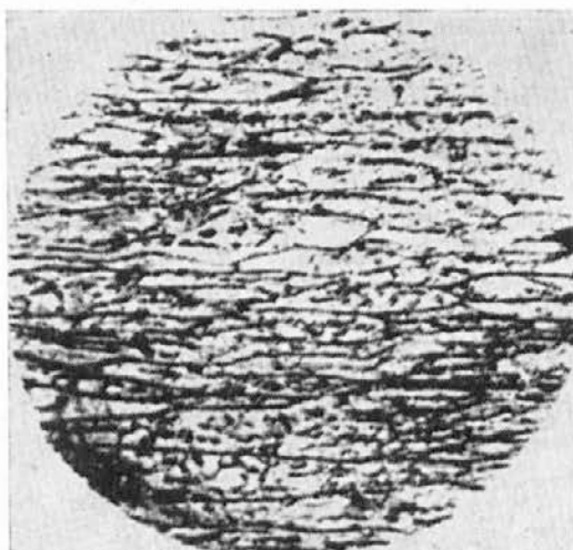
Slika 3 — trakasta struktura Cr-C jekla III X 15 z 1% C in 1,6% Cr. Končna temperatura kovanja je bila 740°C
