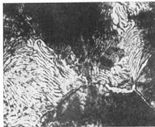
Slika 5a — fina sestava po kovanju pri 1020 do 1050° C, ohlajevano 15° C/min. 500 × povečava
