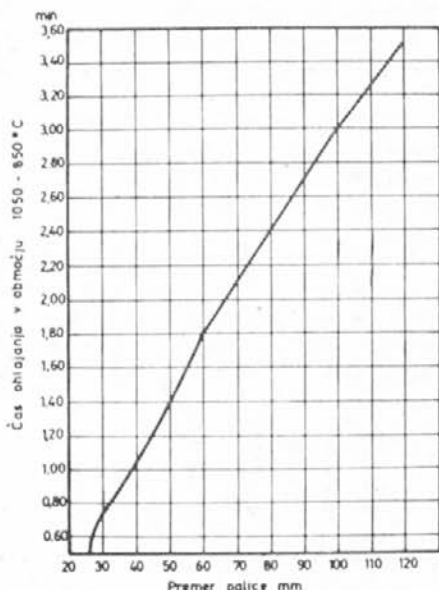
Slika 14 — ohlajevalni čas segretega jekla IXX 15 med toplim prebijanjem 1050—950° C
