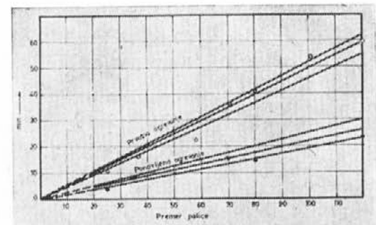
Slika 13 — čas ogrevanja jekla III X 15 v odvisnosti od premera
