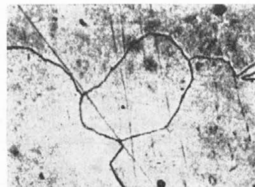
Slika 8 — fina sestava pri 1020 do 1050° C, ohlajevano 75° C/min. Jedkano v natrijevem pikratu, 500 × povečava
