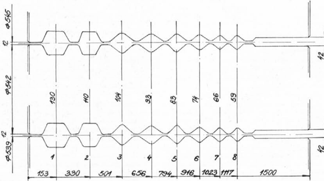
Slika 2 — shema kalibracije II ogrodja — nova varianta
