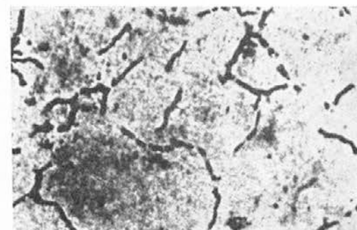
Slika 10 — fina sestava po končanem kovanju pri 920 do 950° C, ohlajevalna hitrost 4° C/min. Jedkanje v natrijevem pikratu, 500 × povečava
