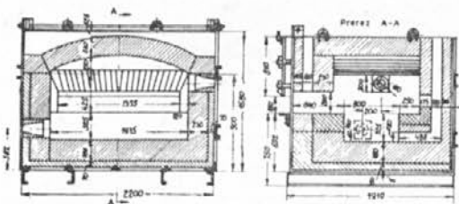
Slika 15 — Muflova peč za ogrevanje palic
