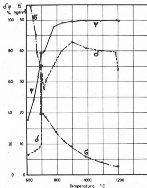
Slika 1 — sprememba mehanskih lastnosti Cr-C jekla z 0,95% C in 1,5% Cr v temperaturnem območju med 600—1200° C
