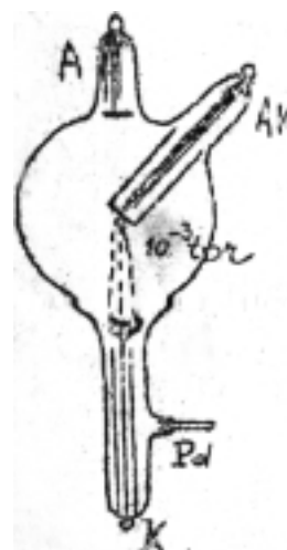
Slika 3: Rentgenska vakuumska elektronka v našem prvem univerzitetnem učbeniku fizike (Peterlin, 1940, 272)
