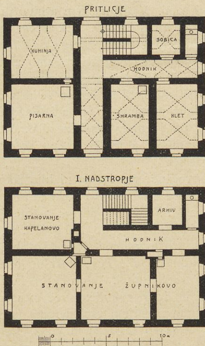
Zupnišče. Tloris.
