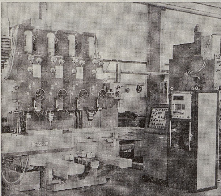
Večvretenski kopirni rezkalni stroj
