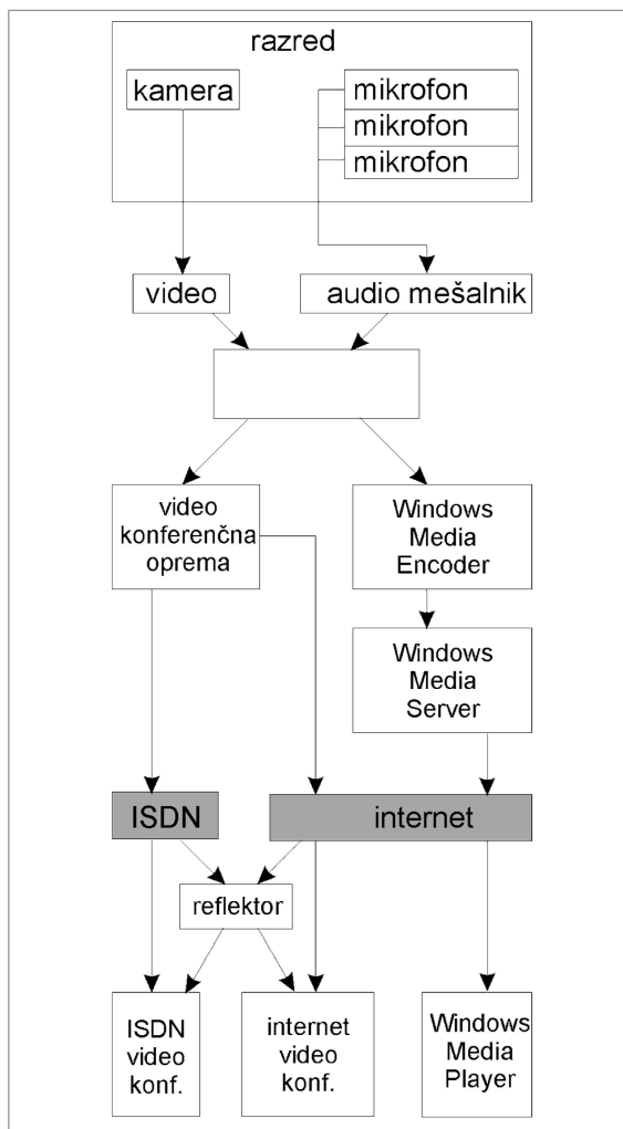
Slika 3: Shema videosistema
