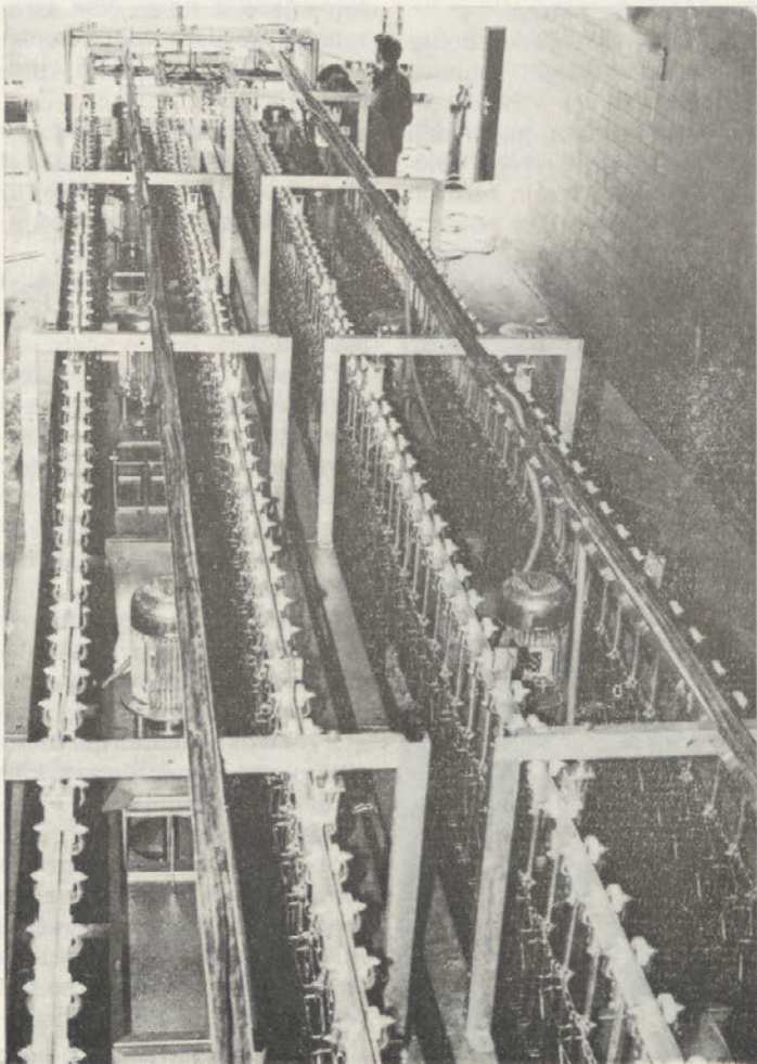
Pogled na novi parilnik
