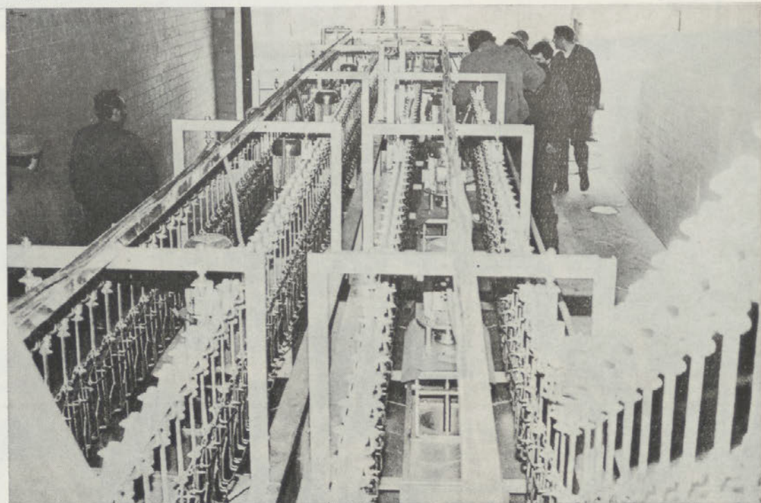
Zaključna dela na parilniku
