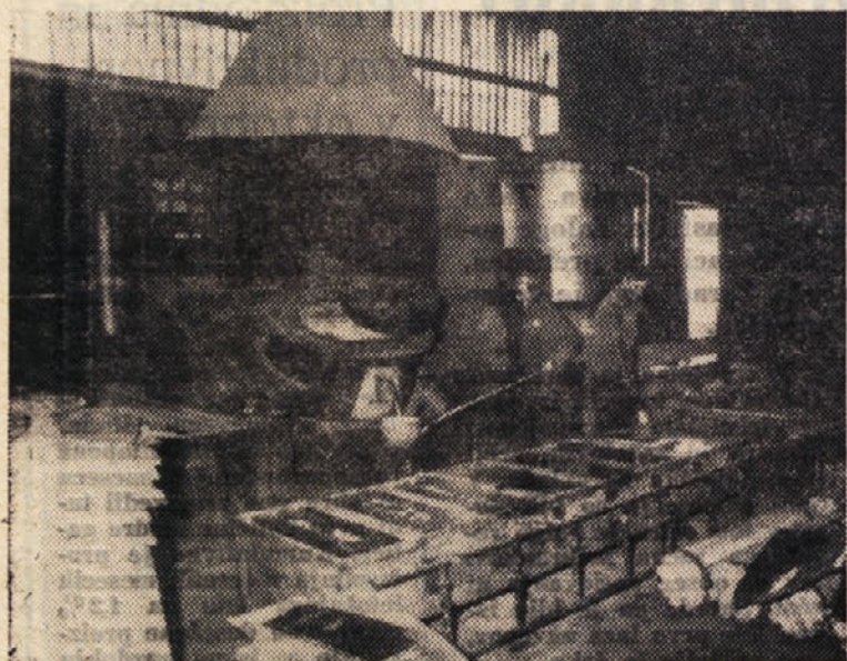
Izlivanje cinka iz električne pretaljevalne peči
