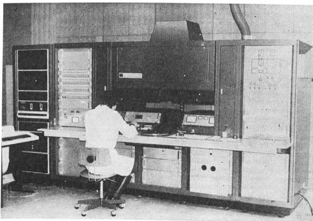
Rentgenski fluorescenčni kvantometer z računalnikom
