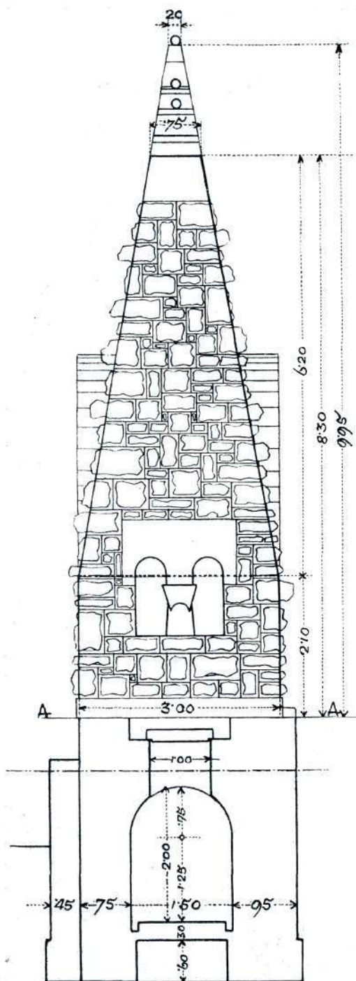
Stransko lice grobnice in prerez grobišča
