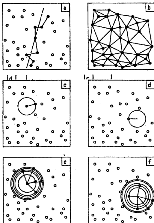
Slika 4: Načini ugotavljanja gostote dreves na osnovi razmika r_1 in r_k
