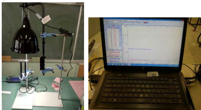
Slika3: Aparatura za merjenje UV sevanja (lasten vir)
