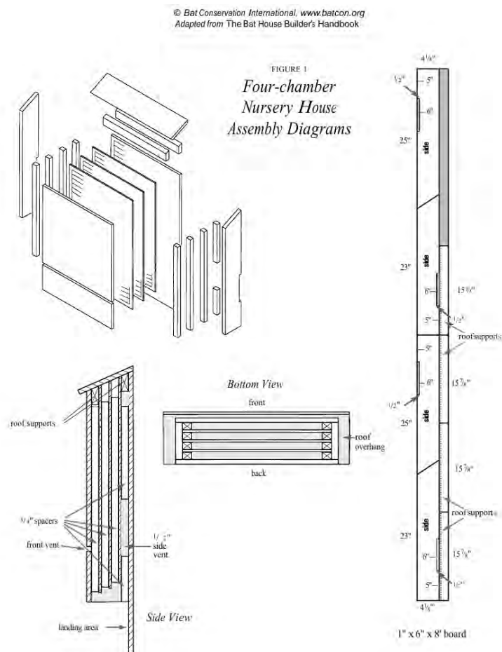
Slika 1: Načrt netopirnice
