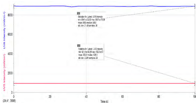
Graf 2: Intenziteta UV sevanja grelne žarnice
