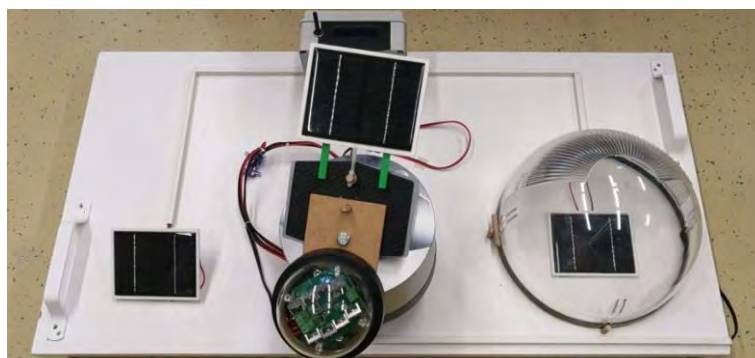
Slika 3: Prenosljiva merilna postaja za merjenje izplena električne energije
