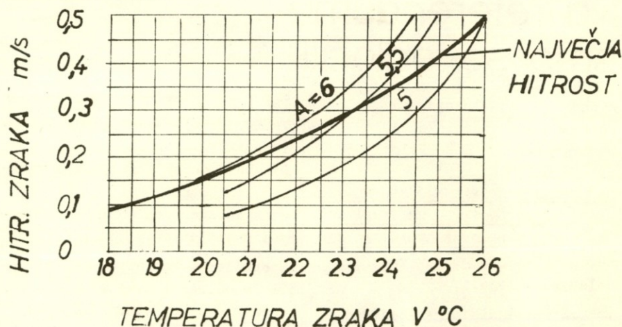
DOPUSTNA HITROST ZRAKA PRI ODPIHAVANJU SEDEČIH OSEB V ODVISNOSTI OD TEMPERATURE ZRAKA
