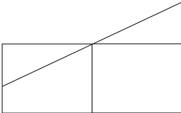
Slika 1: Oresmov diagram.
