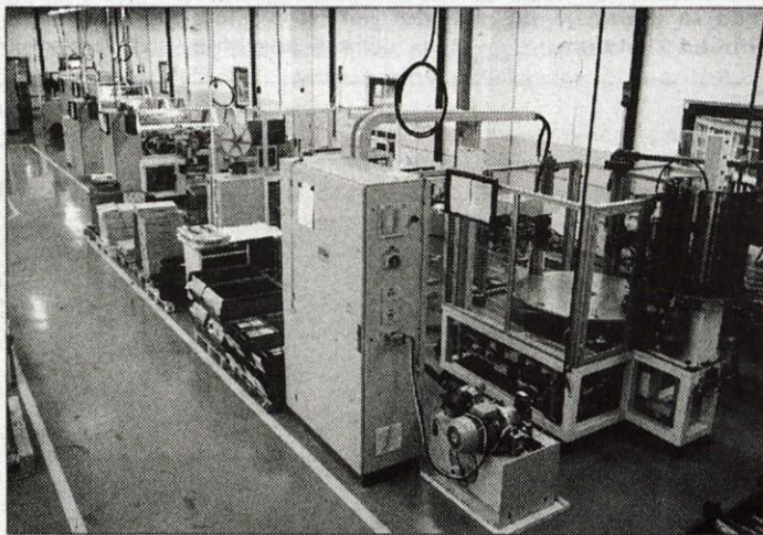
Rotorsko in statorsko proizvodno linijo so kupili pri italijanski firmi Axis, montažno linijo so izdelali sami. Opremo so naročili hkrati z razvojem novega izdelka, naložba je znašala približno milijardo dolarjev.
