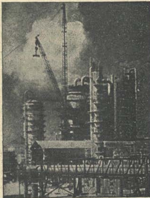
Moderna rafinerija. Velike čistilne naprave, kjer cevi usmerjajo proizvodnjo in predelavo nafte. Nafta teče skozi vrsto naprav, dokler ne dobijo iz nje zaželenih proizvodov (v glavnem bencina).
