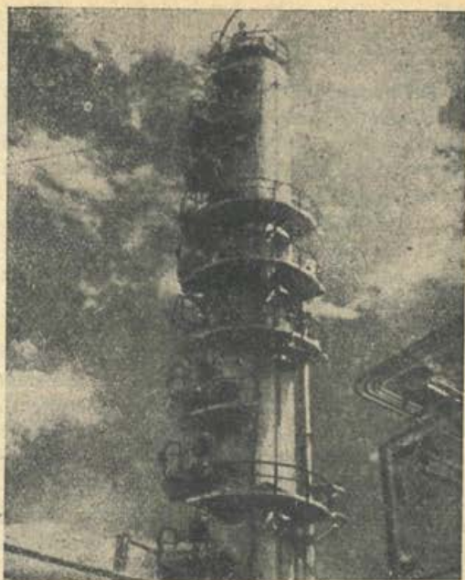
Hladilni stolp sodobne rafinerije. Pri čiščenju nafte potrebujejo veliko vode, zato rafinerij ne zidajo ob najdiščih nafte, temveč ob velikih rekah ali ob morju. Za tono nafte je treba 15–18 ton vode.
