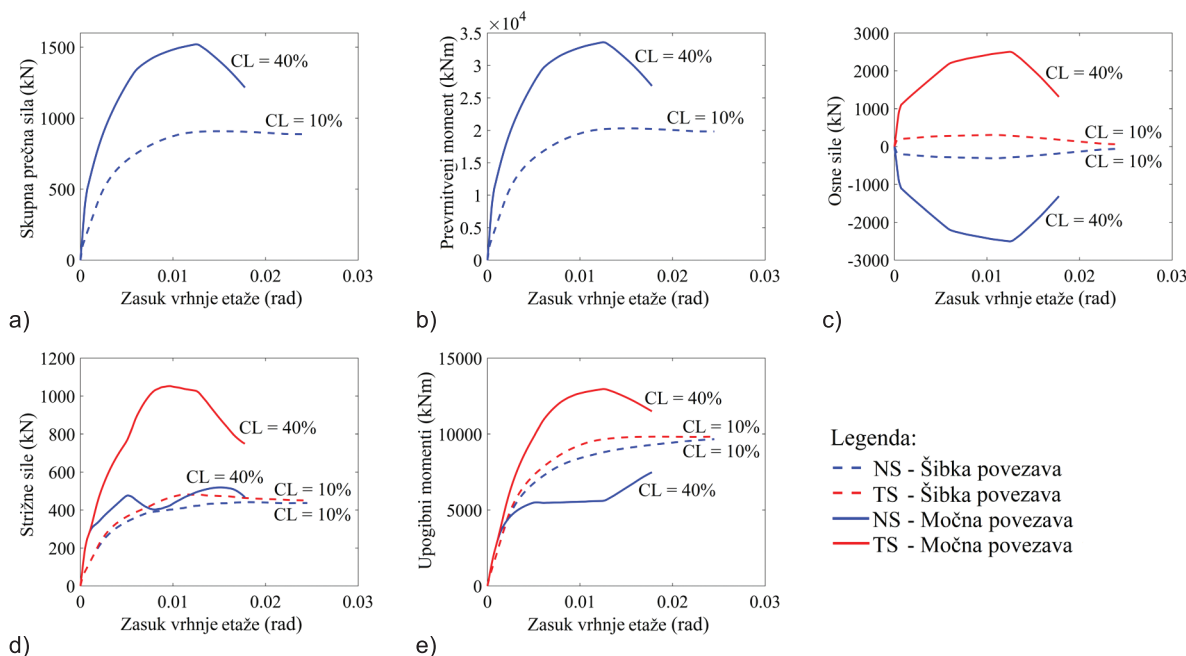
Slika 5. Zveza med a) skupno prečno silo, b) prevrtnitvenim momentom, c) osnimi silami v stenah ki so posledica potresne obtežbe, d) prečnimi silami v stenah ter e) upogibnimi momenti v stenah in zasukom vrhnje etaže.
