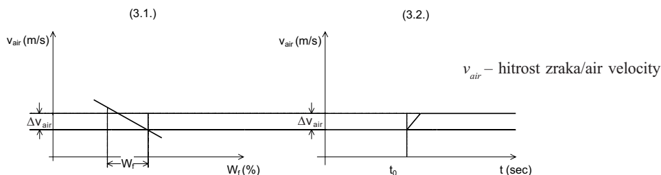
Sl. 3. Ustajene in dinamične lastnosti hitrosti osuševalnega zraka Fig. 3. Static and dynamic properties of the velocity of the drying air
