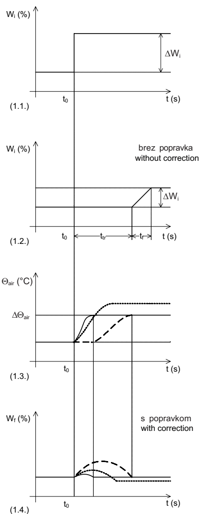
Sl. 1. Dinamične lastnosti Fig. 1. Dynamic properties
