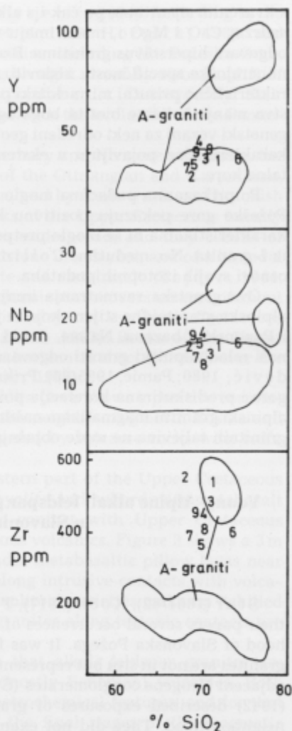
Sl. 8. Varijacioni dijagrami za Y, Nb i Zr u odnosu na SiO 2 za A-granite (Collins et al., 1982)
