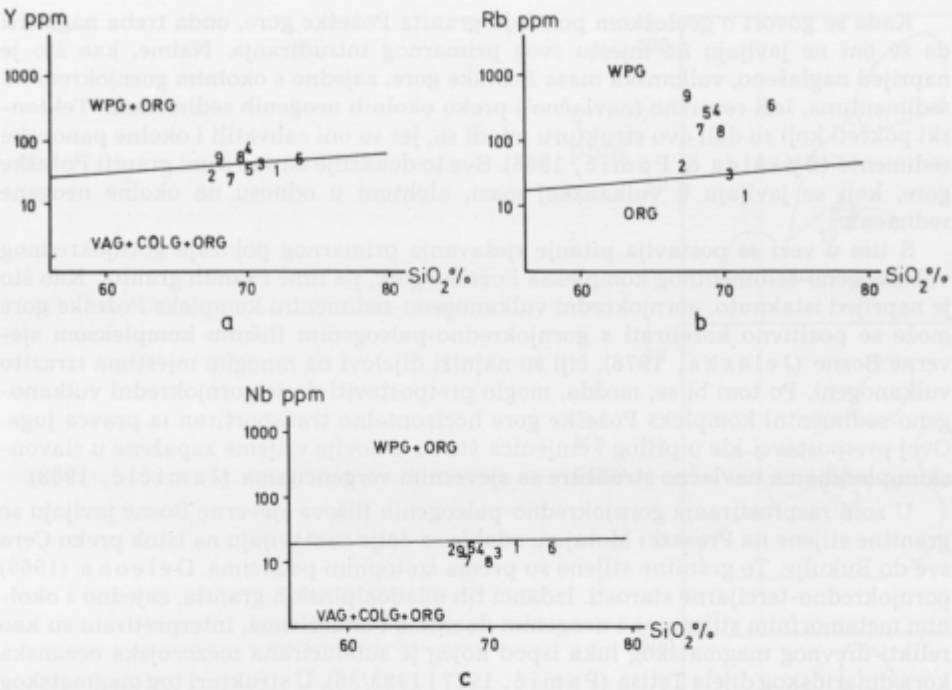
Sl. 6. Varijacioni dijagrami za Y (a), Rb (b) i Nb (c) u odnosu na SiO 2 (Pearce et al., 1984)
